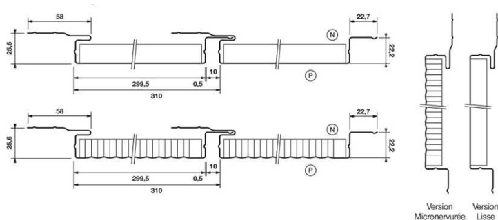
Profil des lames IROISE 300 bordées joints creux
