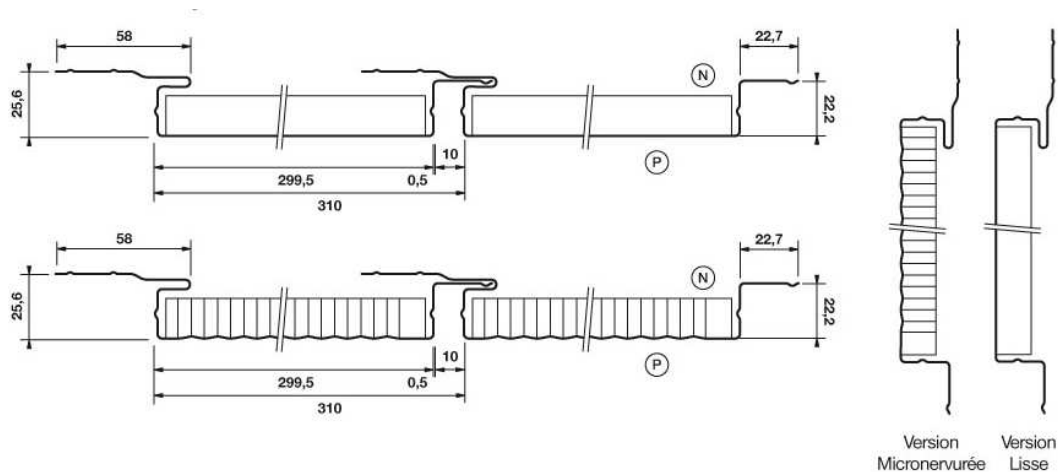
Figure 07.1 - Lame IROISE 300 bordée avec emboîtement joint creux – largeur utile 310
