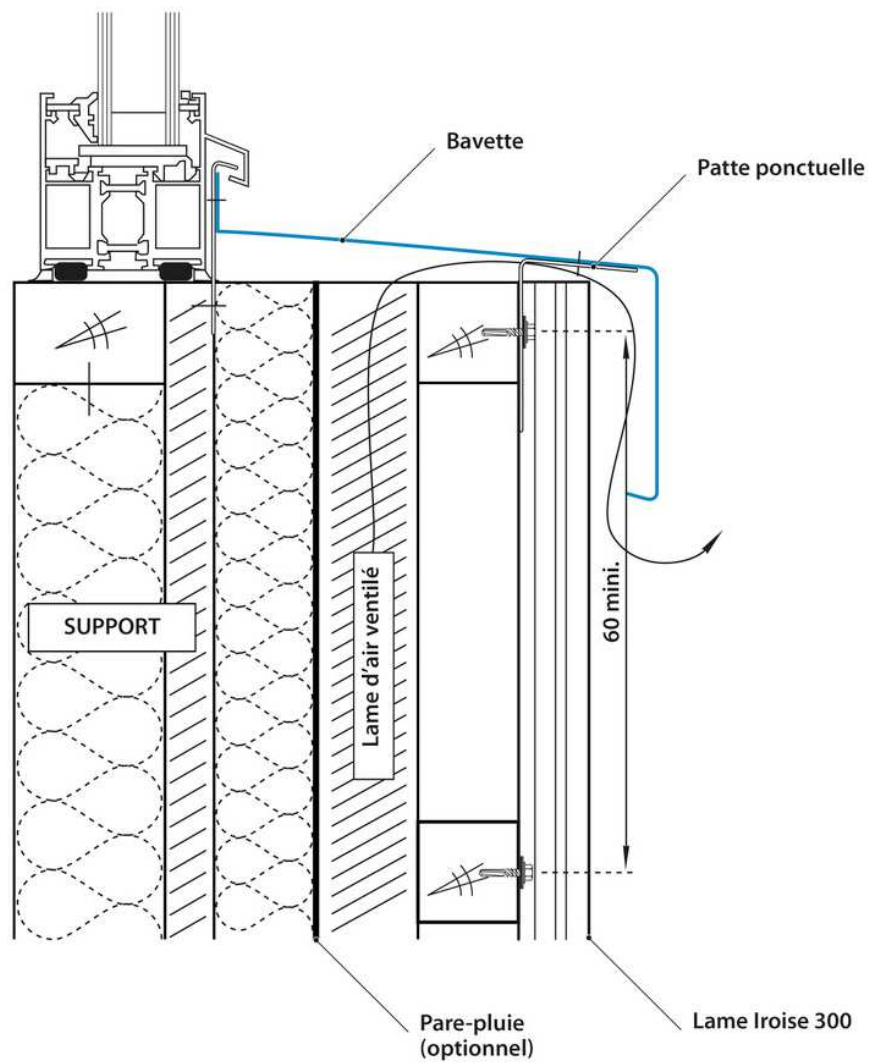
Figure 30 C-1 -Détails appui (pose COB et CLT)
