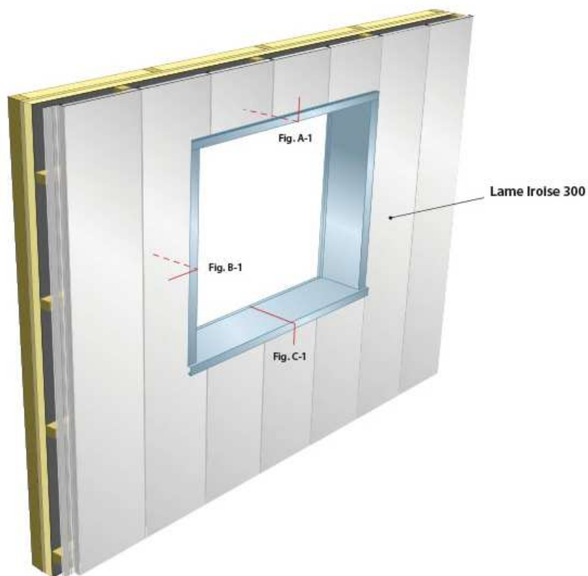
Figure 29 – Encadrement ouvertures pour COB et CLT
