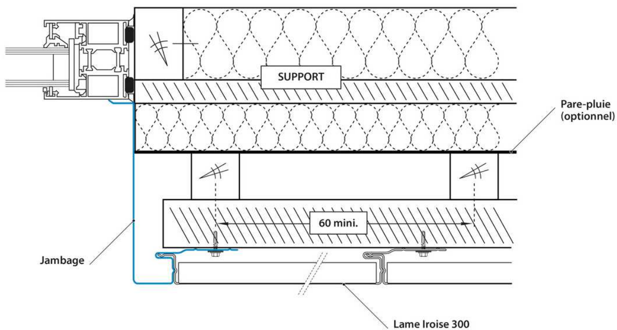
Figure 30 B-1 -Détails jambage (pose COB et CLT)
