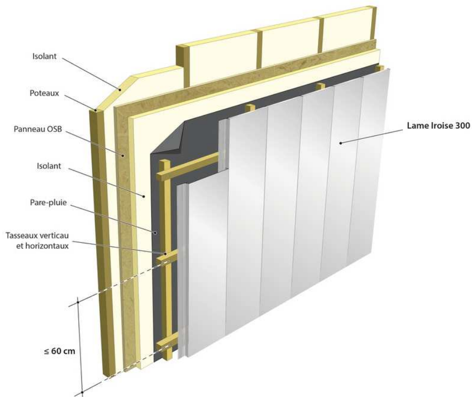
Figure 28 – Principe de pose pour COB et CLT
