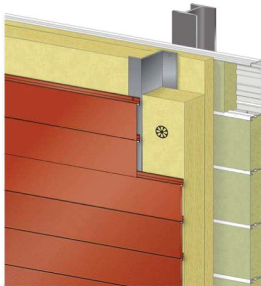
Principe de pose en double peau : bardage horizontal
