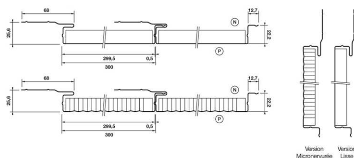
Profil des lames IROISE 300 bordées joints serrés
