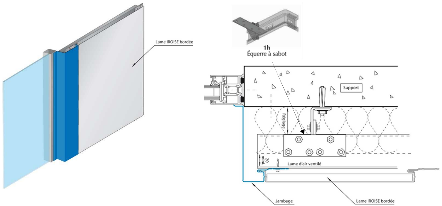
Figure 15 – Détails jambage pose verticale
