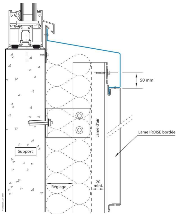
Figure 13 – Détail appui 2
