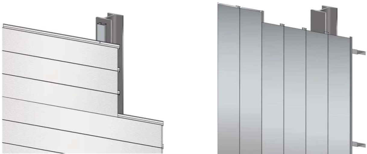
Principe de pose en simple peau : bardage horizontal à gauche et bardage vertical à droite
