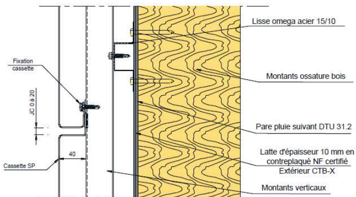
COUPE A-A
