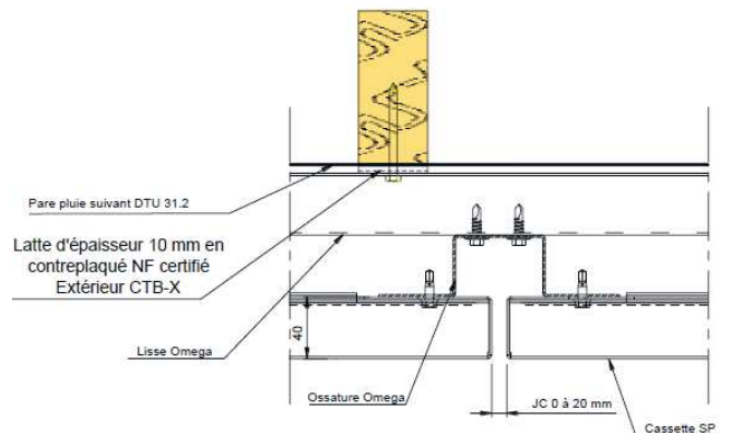
COUPE B-B
