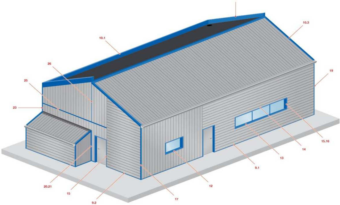
Figure 08.2 – Repérage des détails GLENAN
