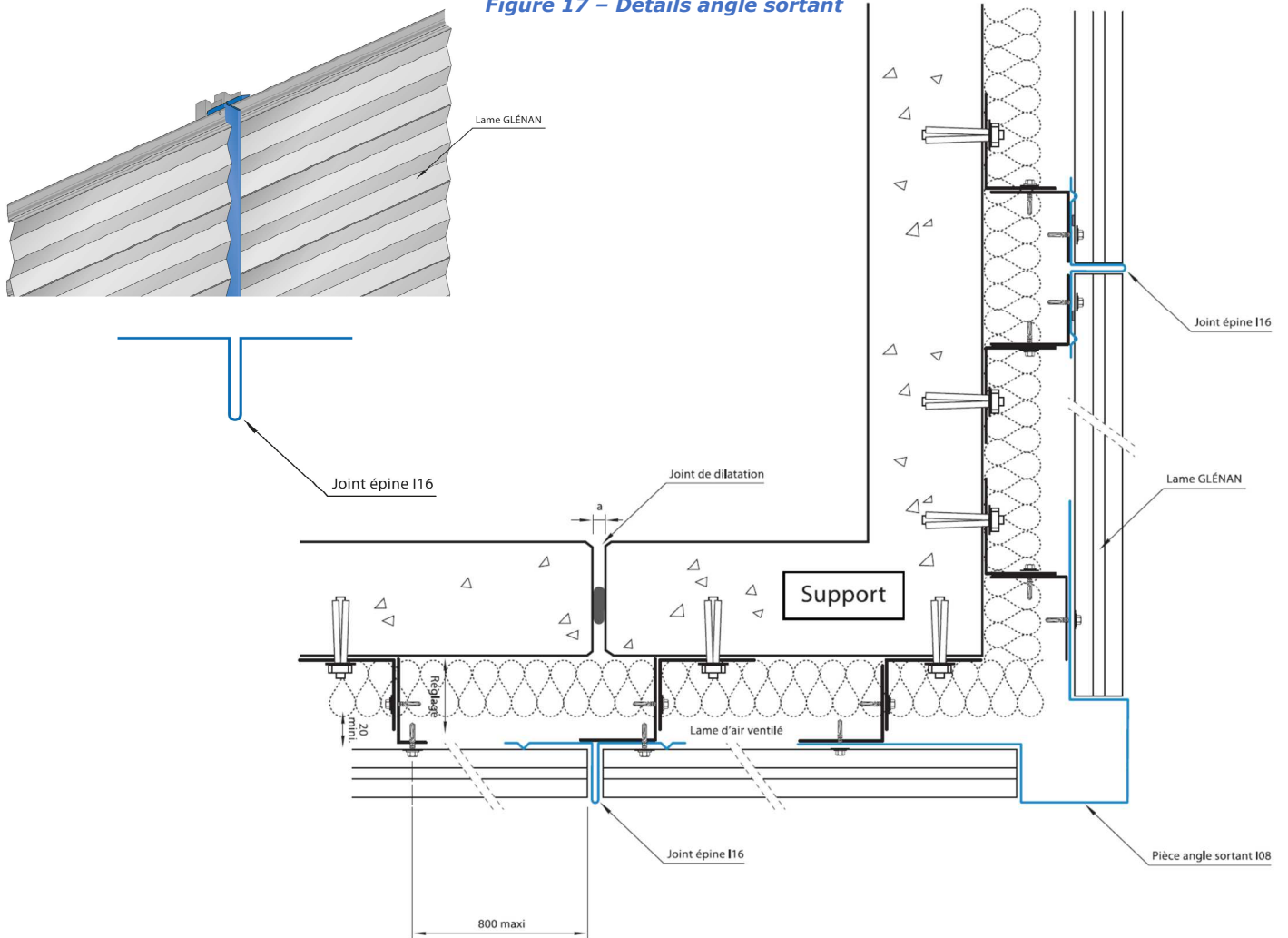
Figure 17.1 Détails joint épine, pose horizontale
