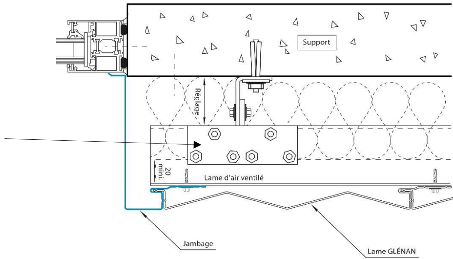
Figure 15 – Détails jambage pose verticale
