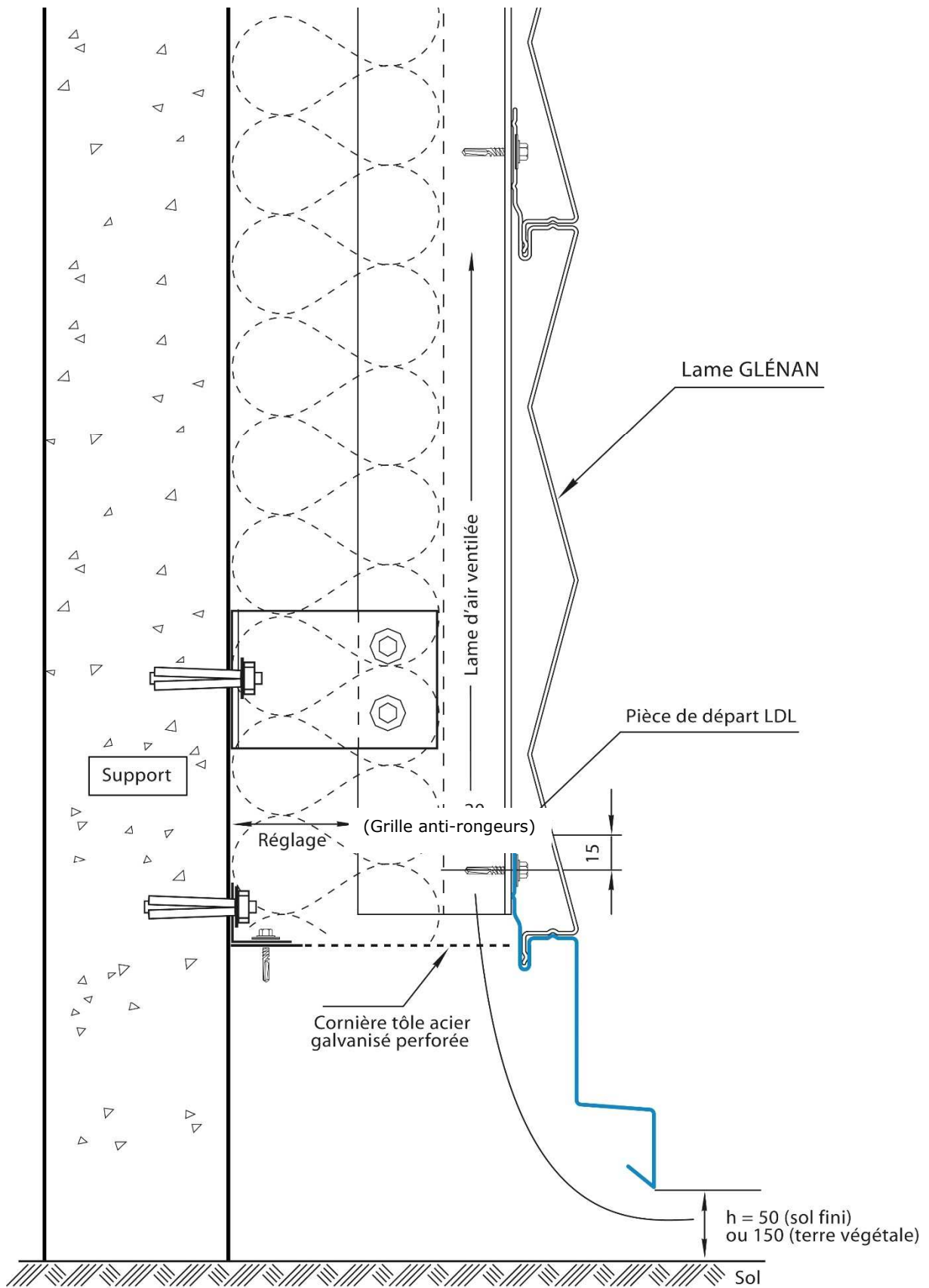
Figure 09.3 – Pièce de départ 2 – LDL
