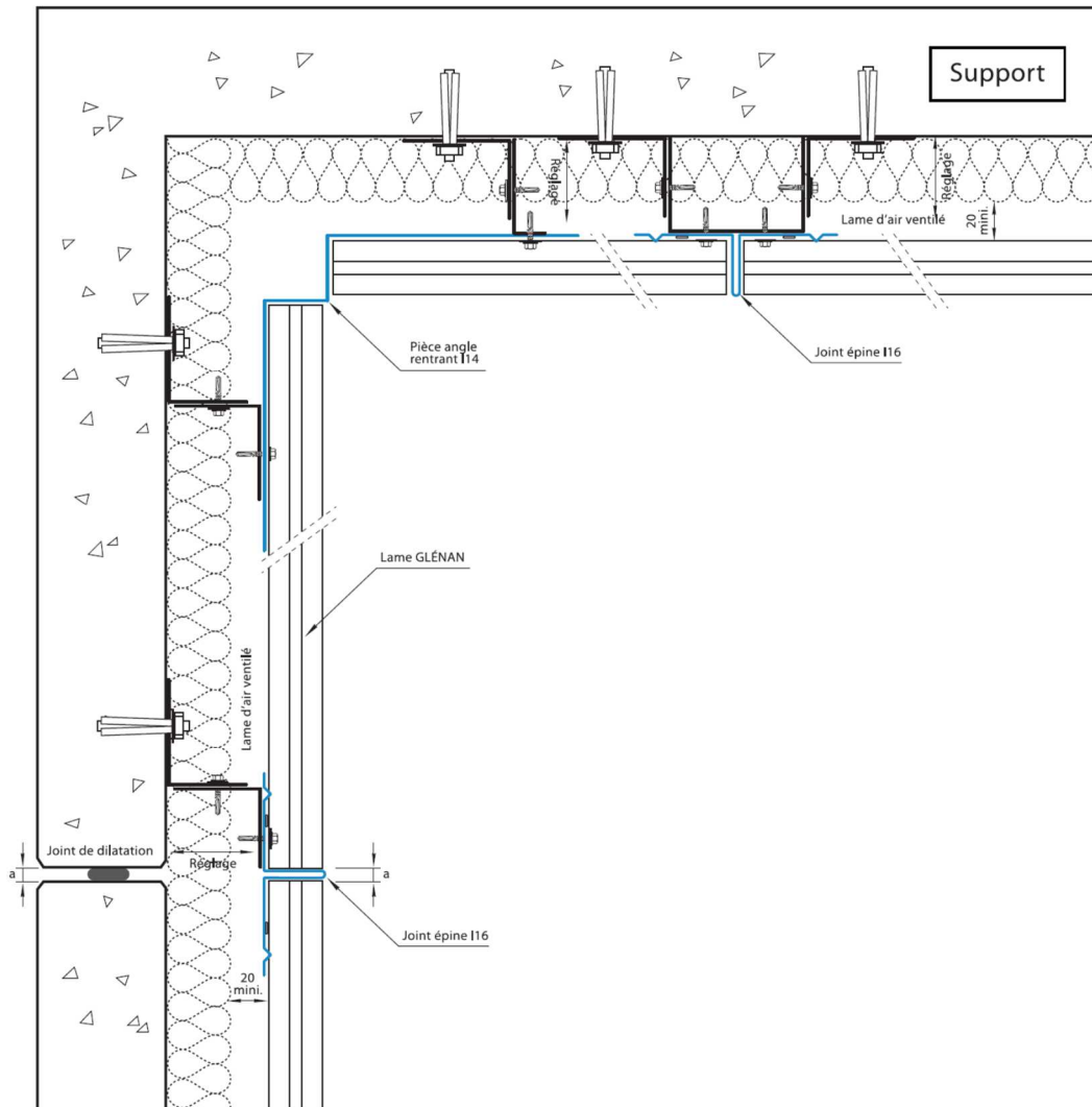
Figure 20 – Détails angle rentrant 1 Pose horizontale
