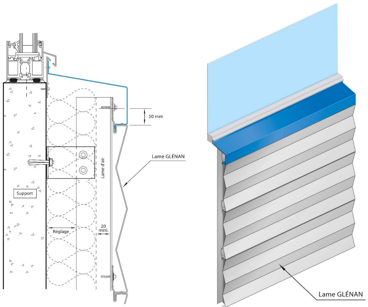
Figure 13 – Détail appui 2
