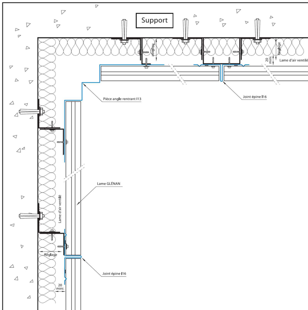
Figure 21 – Détails angle rentrant 2 Pose horizontale
