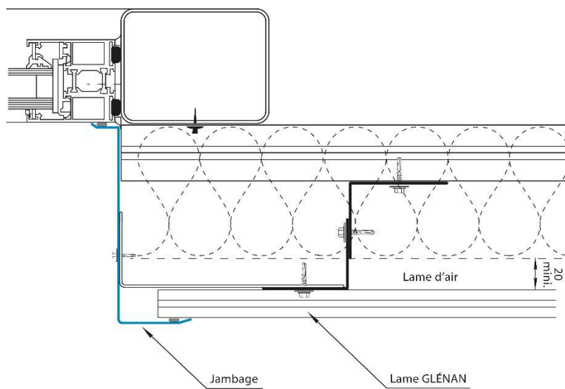
Figures 16.1 et 16.2 – Détails jambage pose horizontale
