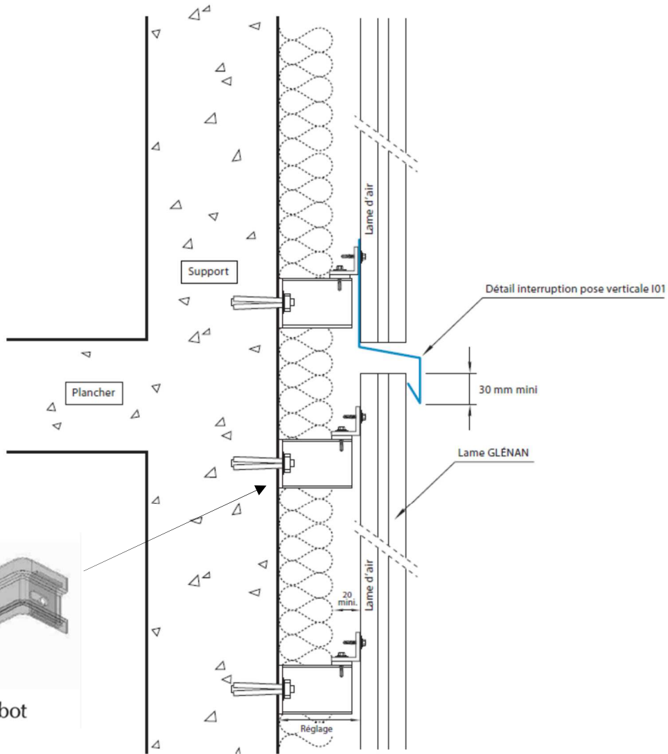
Figure 25 – Détail fractionnement pose verticale
