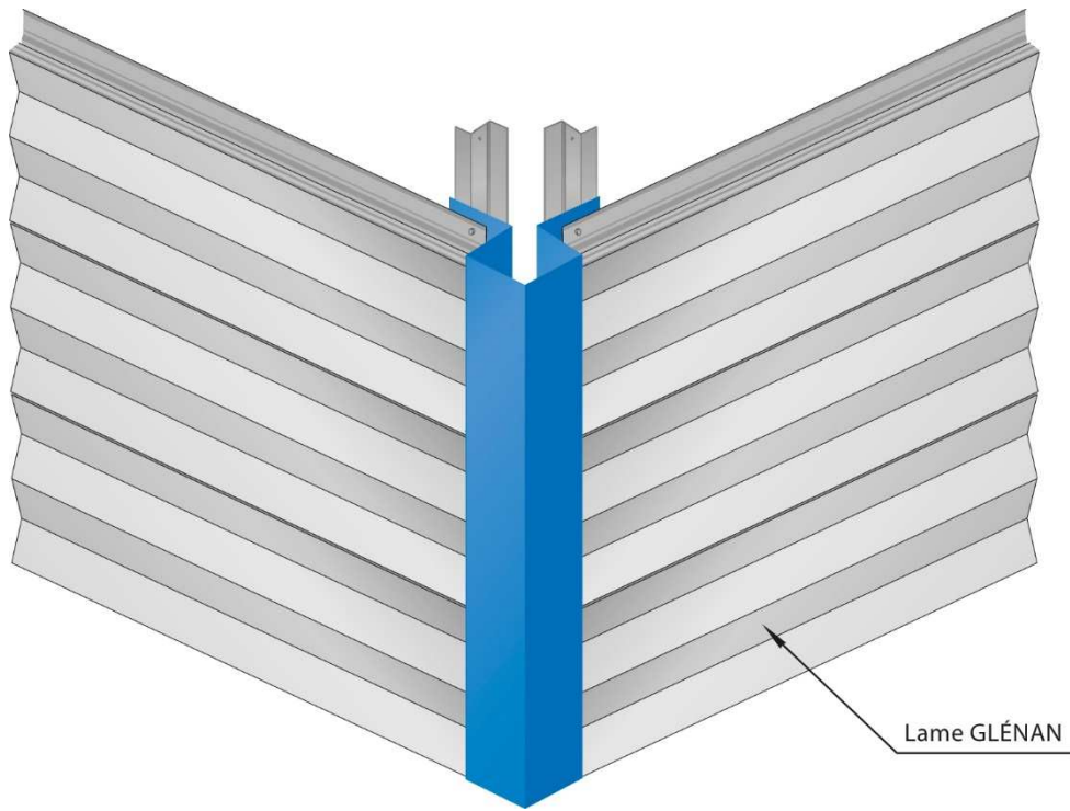
Figure 17 – Détails angle sortant
