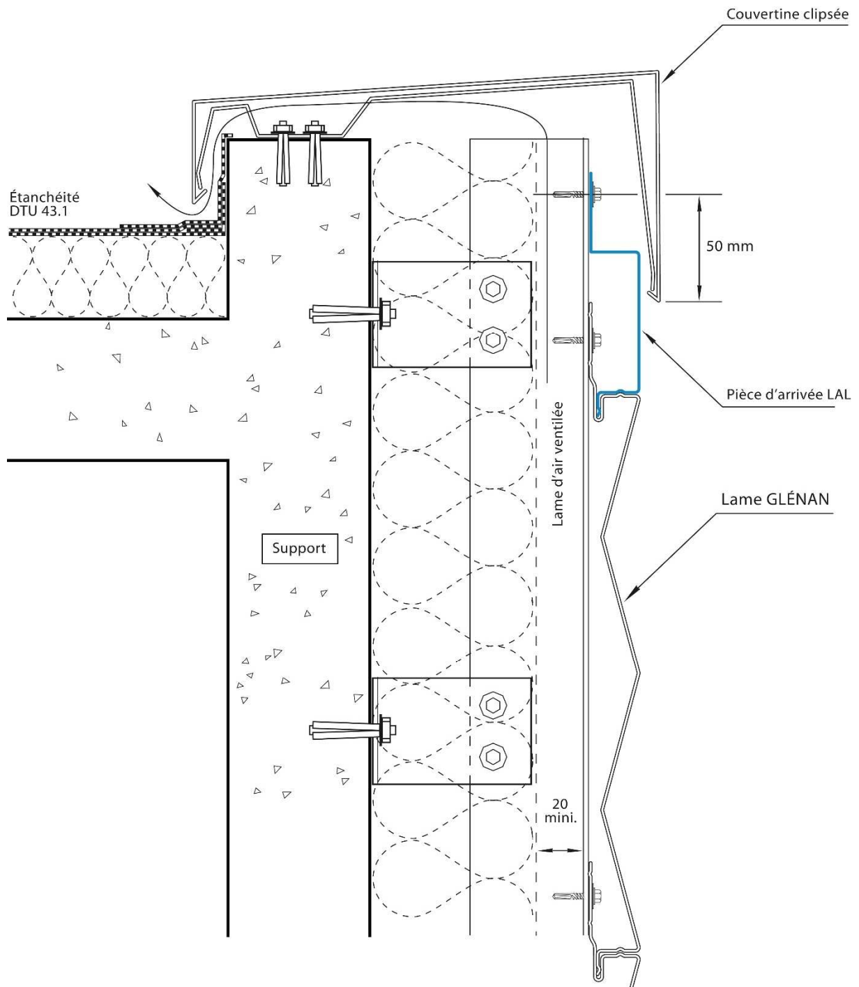
Figure 10 – Détail acrotère 1 LAL et ventilation haute
