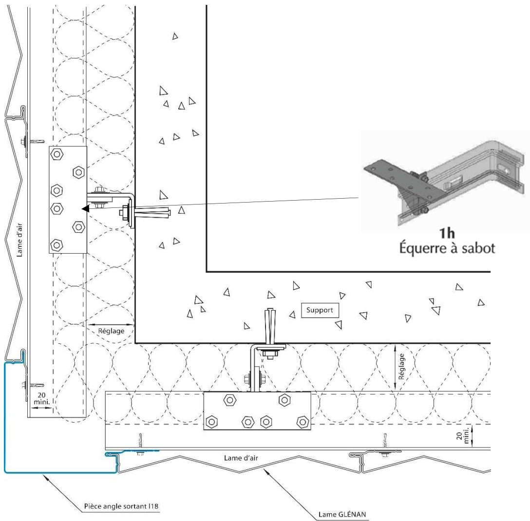
Figure 23 – Détail angle sortant pose verticale
