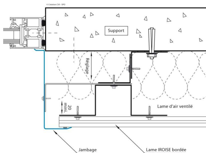
Figure 16 – Détails jambage pose horizontale
