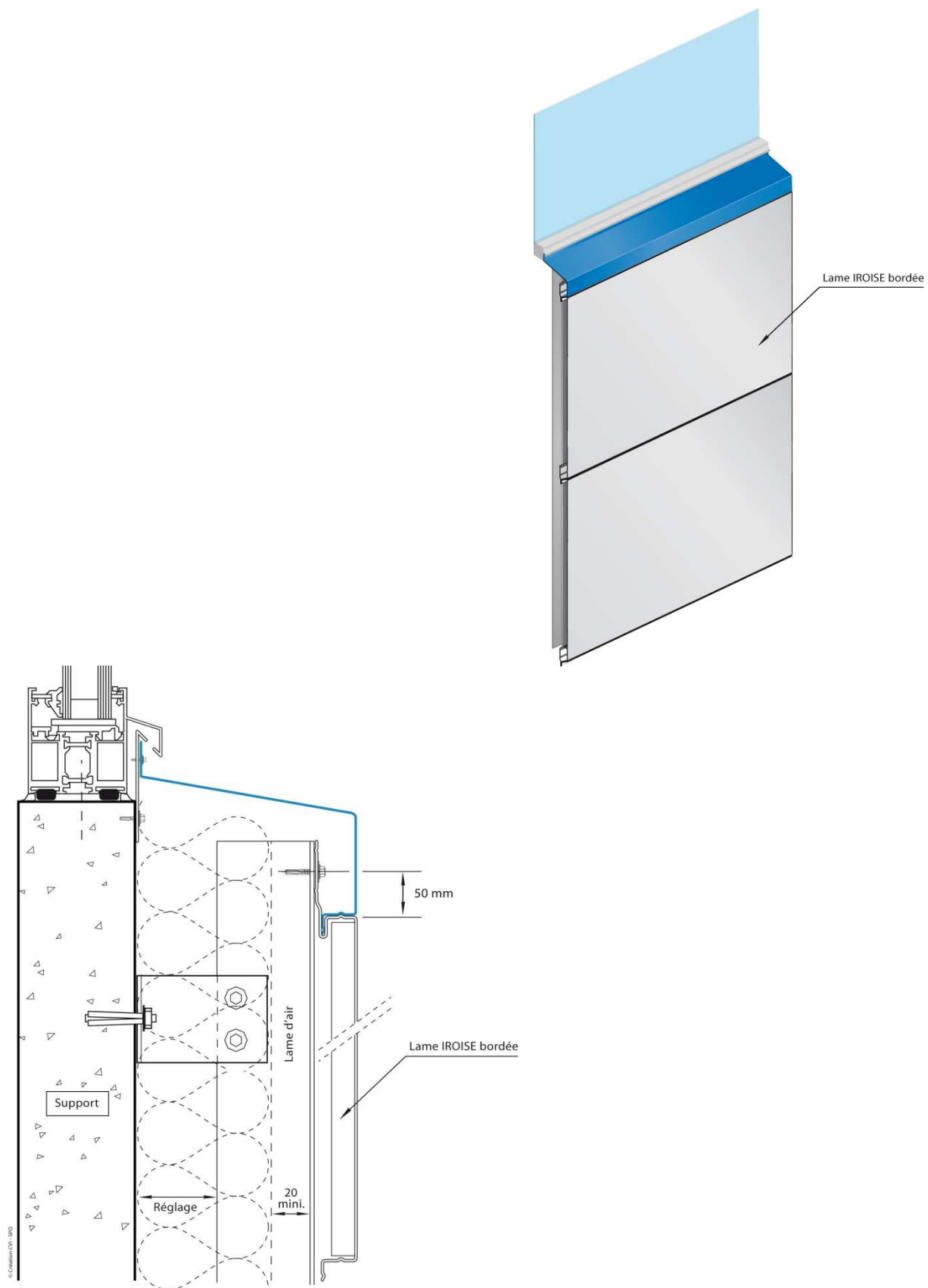
Figure 13 – Détail appui 2
