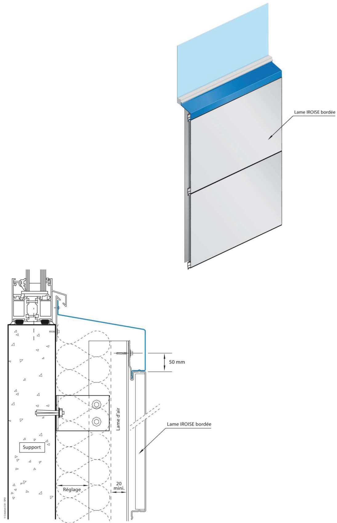
Figure 13 – Détail appui 2 en pose horizontale
