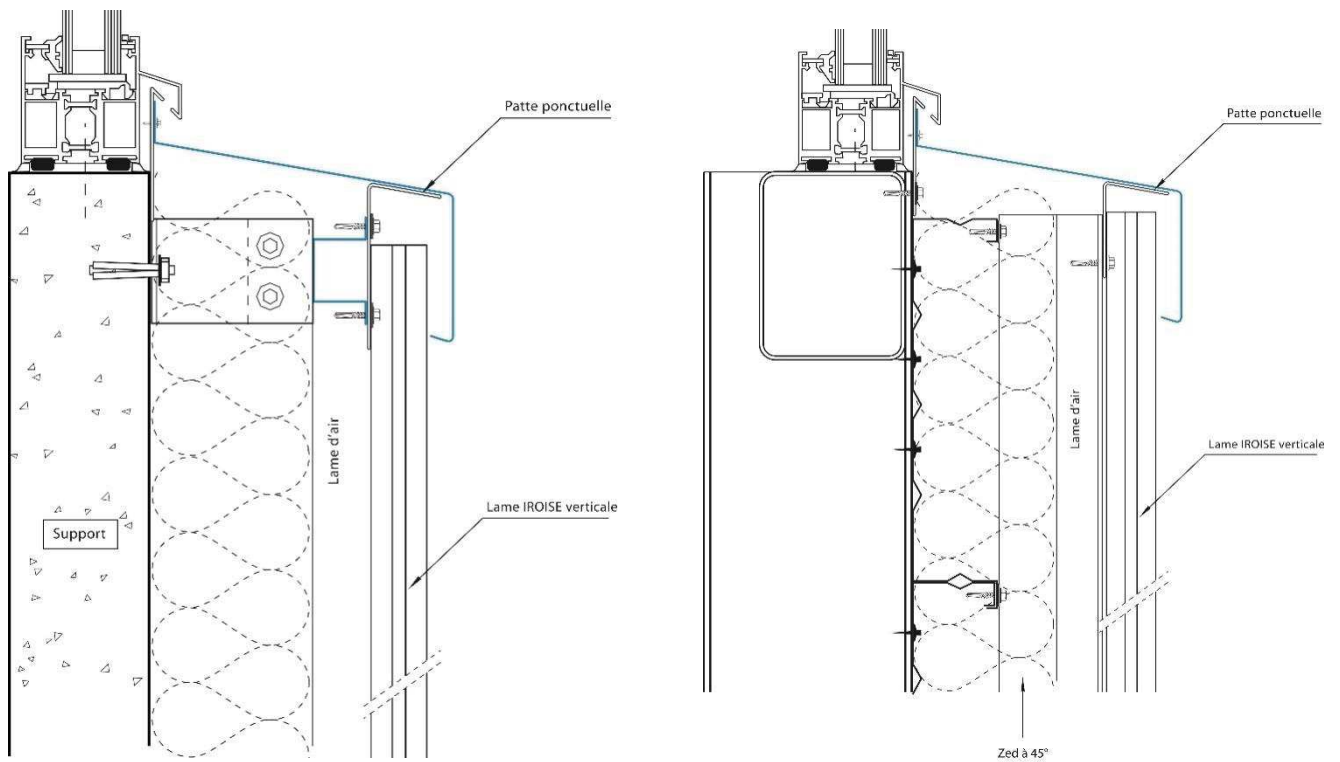
Figure 12a et b – Détail appui 1 : pose rapportée (a) et pose en double peau (b) en pose verticale
