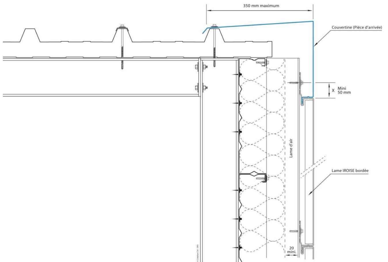
Figure 10.3 – Détail acrotère 3 Coiffe avec panneaux sandwichs
