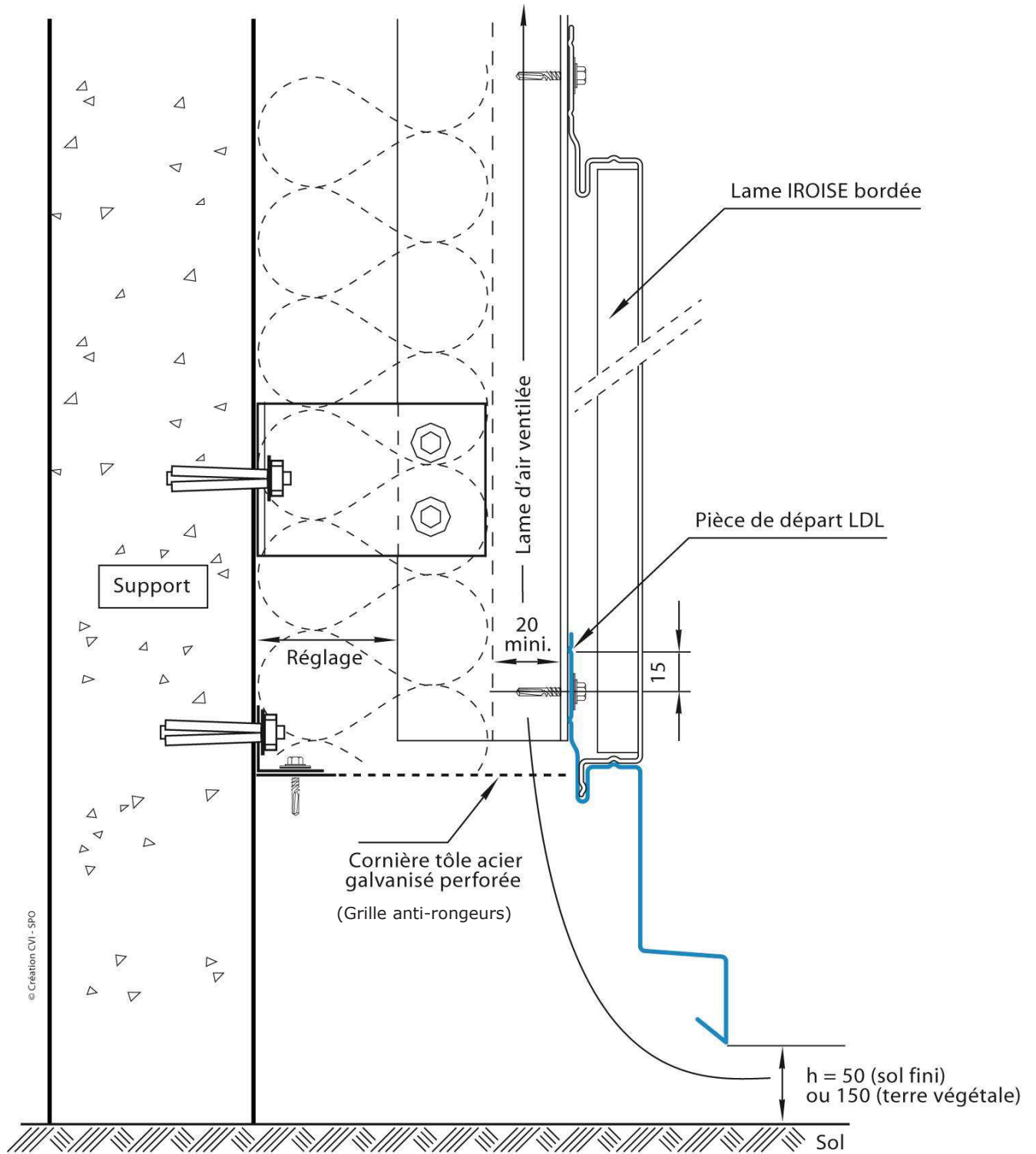
Figure 09.3 – Pièce de départ 2 – LDL
