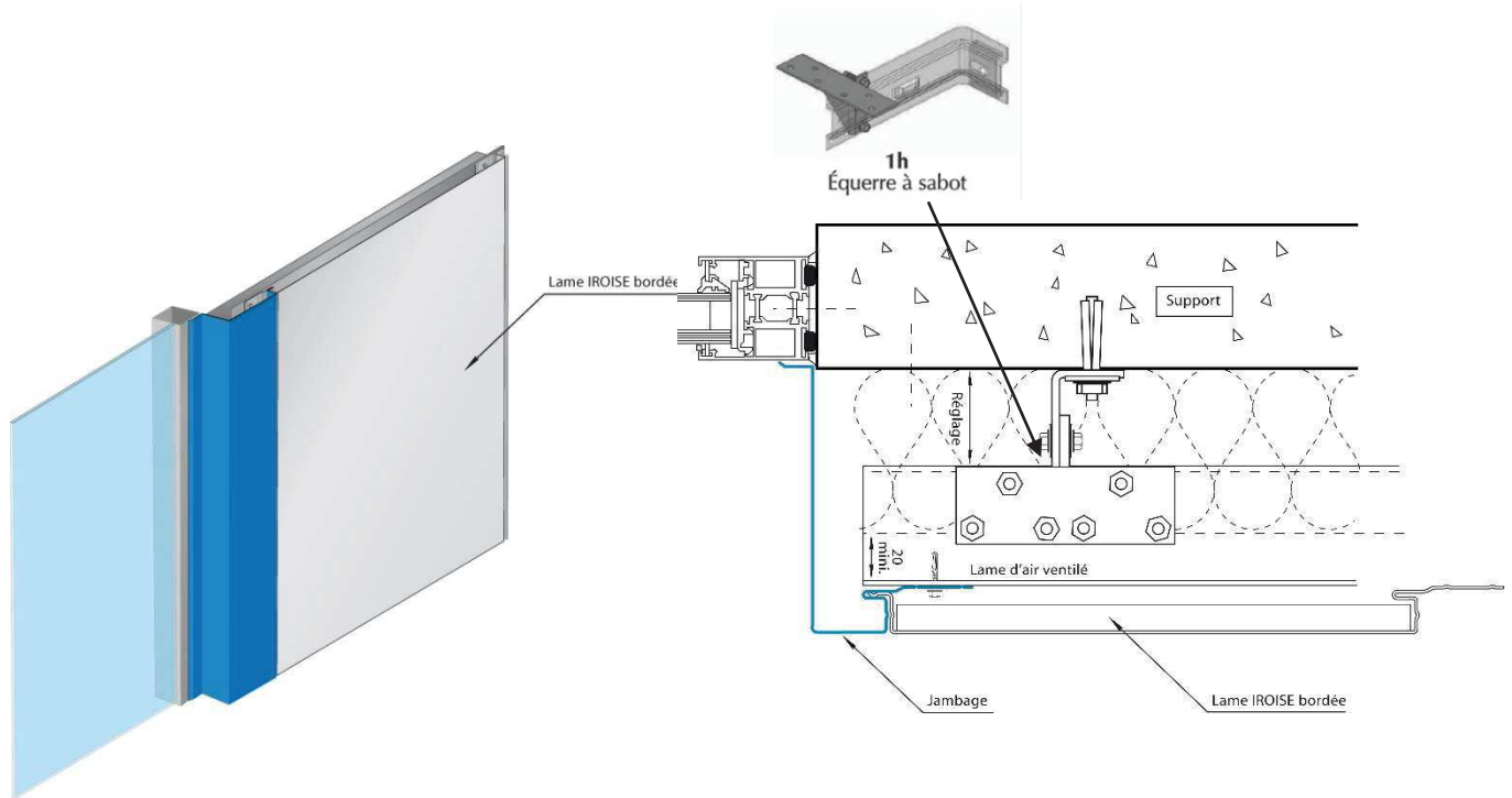
Figure 15 – Détails jambage pose verticale
