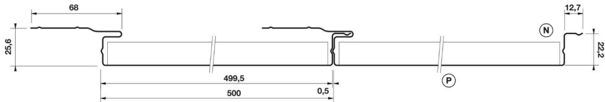
Figure 08.2 - Lame IROISE 500 bordée avec emboîtement joint serré - largeur utile 500
