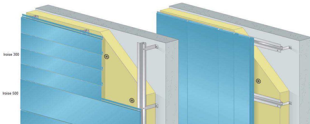
Principe de pose en bardage rapporté : bardage horizontal à gauche et bardage vertical à droite
