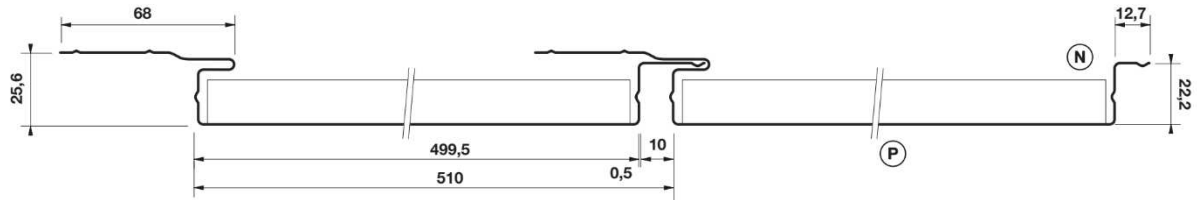
Figure 08.1 - Lame IROISE 500 bordée avec emboîtement joint creux - largeur utile 510
