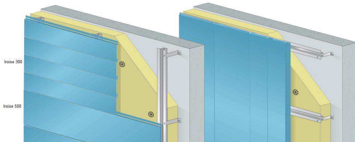
Figure 08.3c et d – Types de pose des lames IROISE 500 bordées
