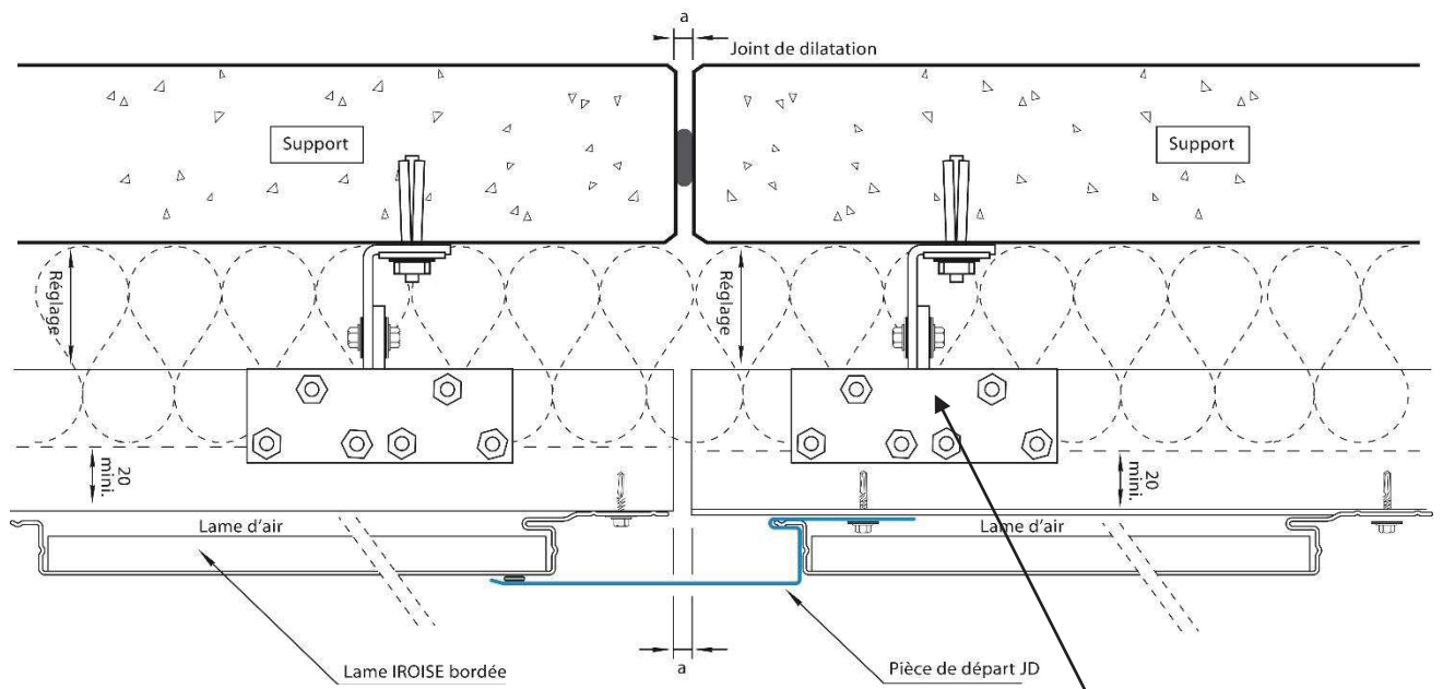
Figure 26 – Détail joint de dilatation pose verticale
