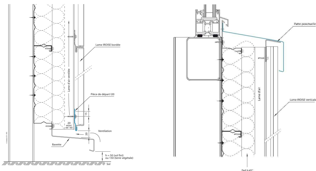
Principe de pose en double peau : bardage horizontal à gauche et bardage vertical à droite
