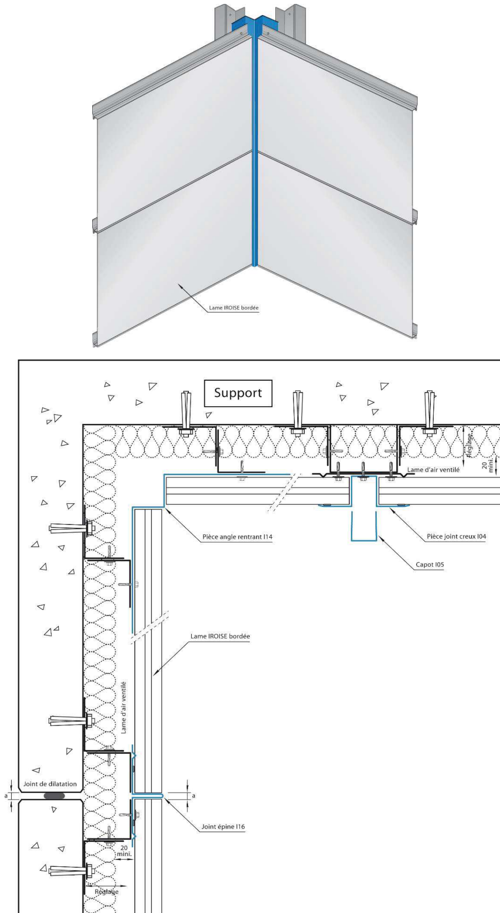
Figure 20 – Détails angle rentrant 1 Pose horizontale
