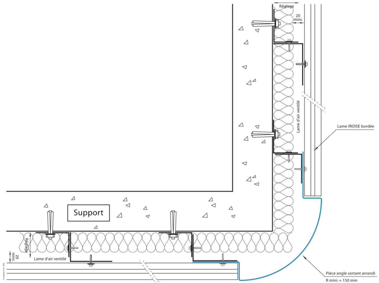
Figure 18 – Détails angle sortant arrondi
