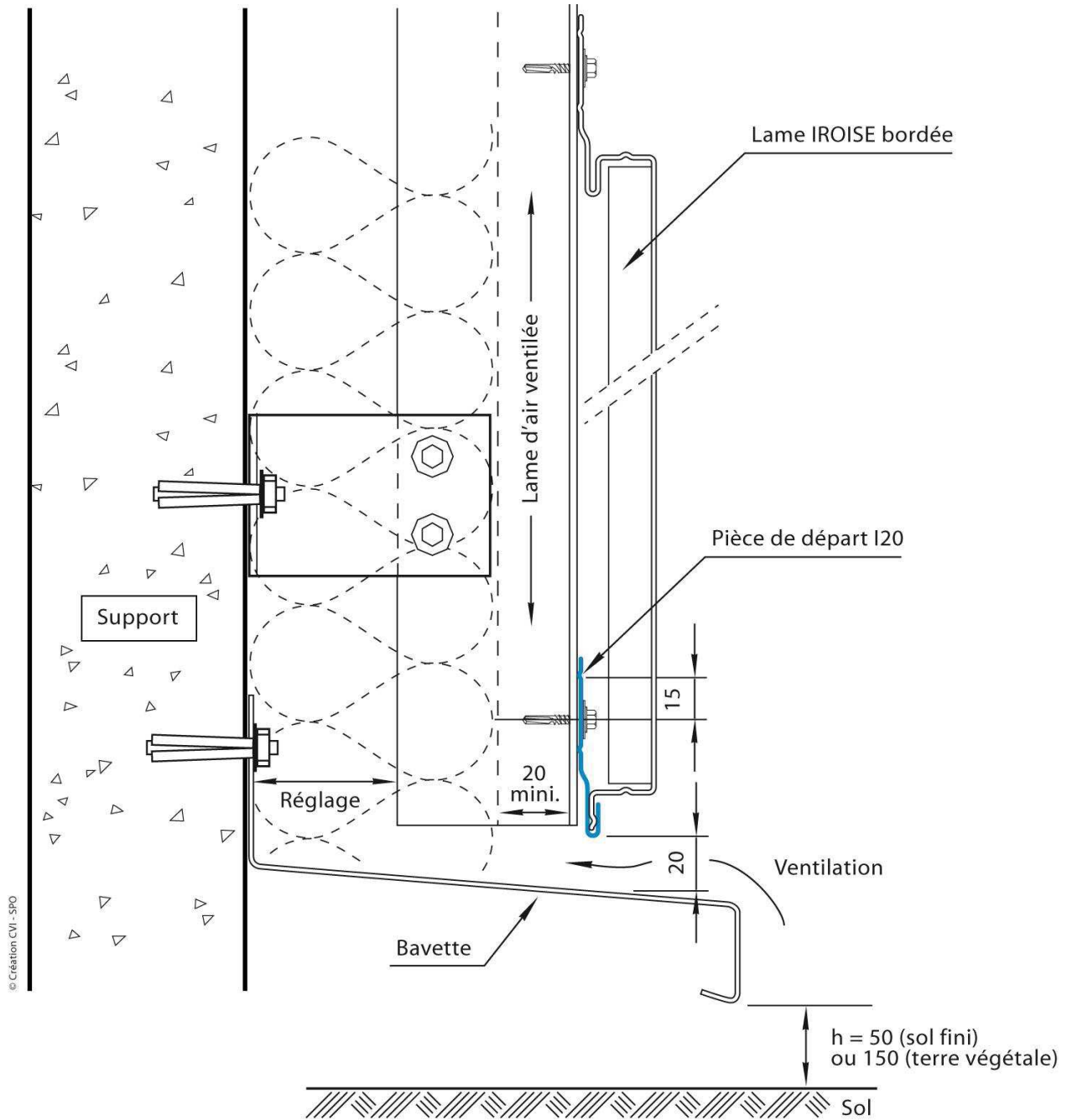
Figure 09.1 – Pièce de départ 1 - I20 (pose rapportée)
