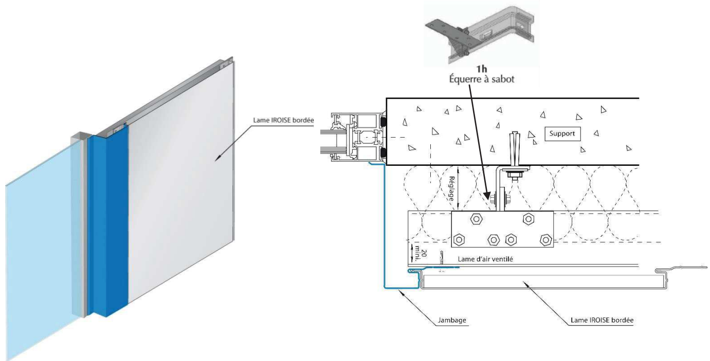
Figure 15 – Détails jambage pose verticale
