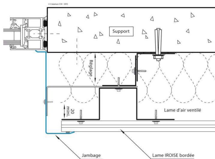
Figure 16 – Détails jambage pose horizontale
