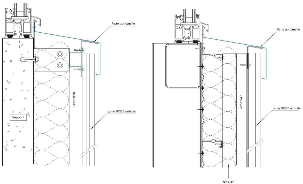
Figure 12 a et b – Détail appui 1 : pose rapportée (a) et pose en double peau (b) en pose verticale
