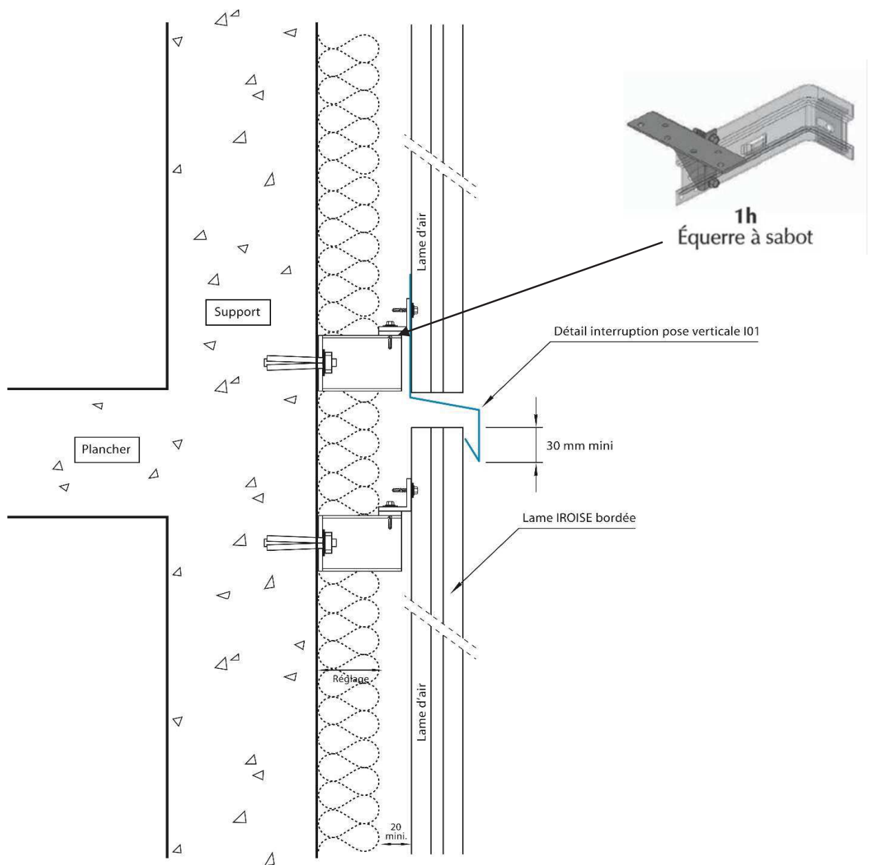
Figure 25 – Détail fractionnement pose verticale
