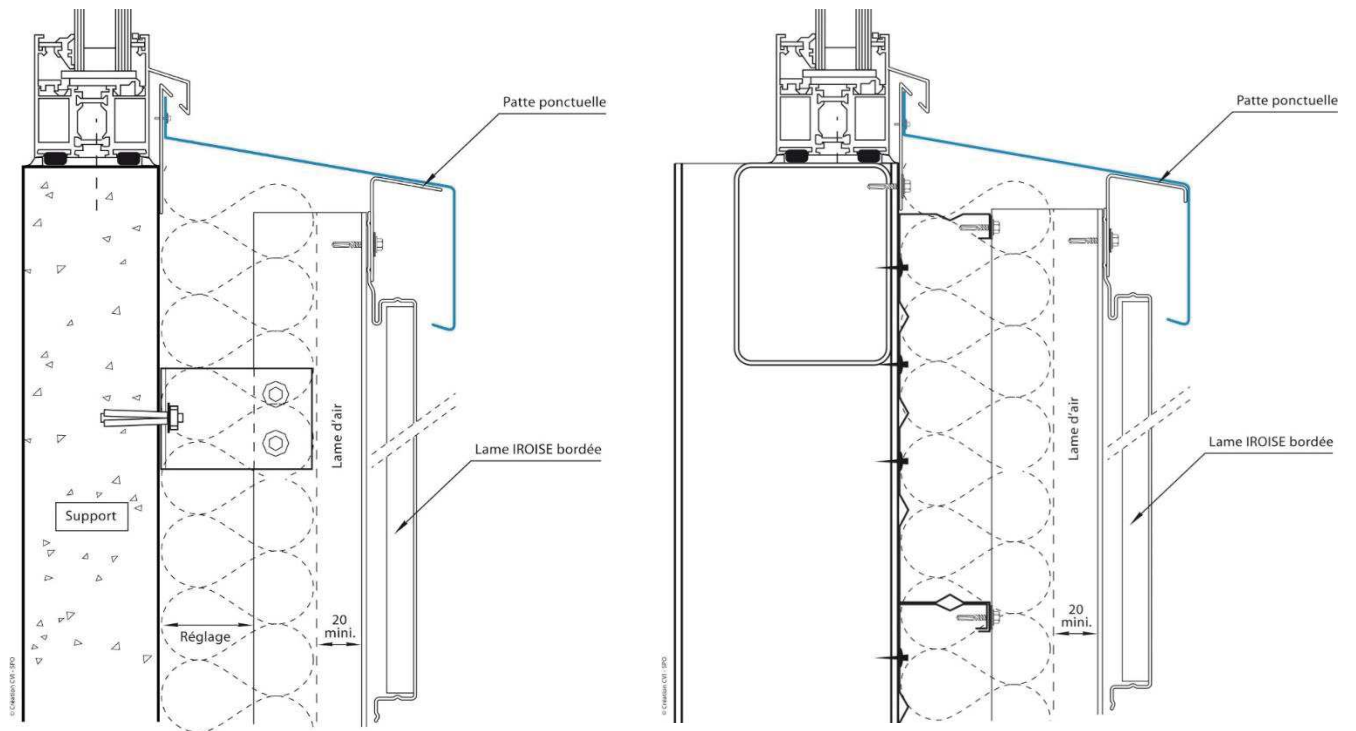
Figure 12 – Détail appui 1 : pose rapportée et pose en double peau en pose horizontale
