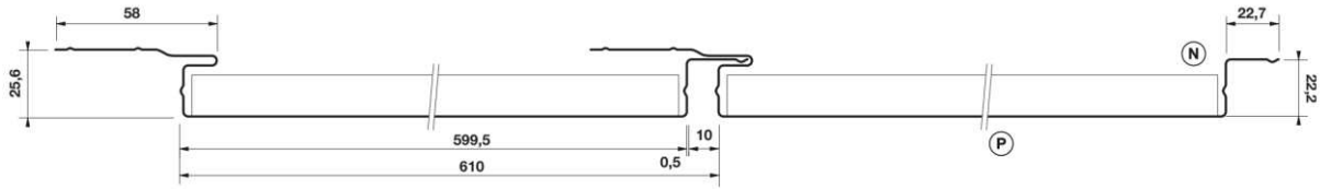
Figure 07.1 - Lame IROISE 600 bordée avec emboîtement joint creux - largeur utile 510
