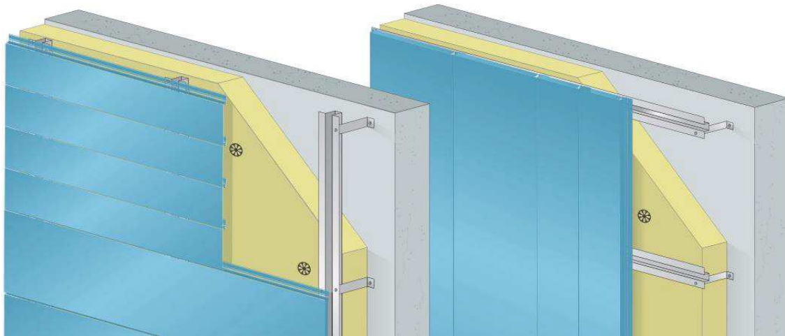
Figure 08.1c et d – Types de pose des lames IROISE 600 bordées
