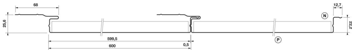
Figure 07.2 - Lame IROISE 600 bordée avec emboîtement joint serré - largeur utile 600
