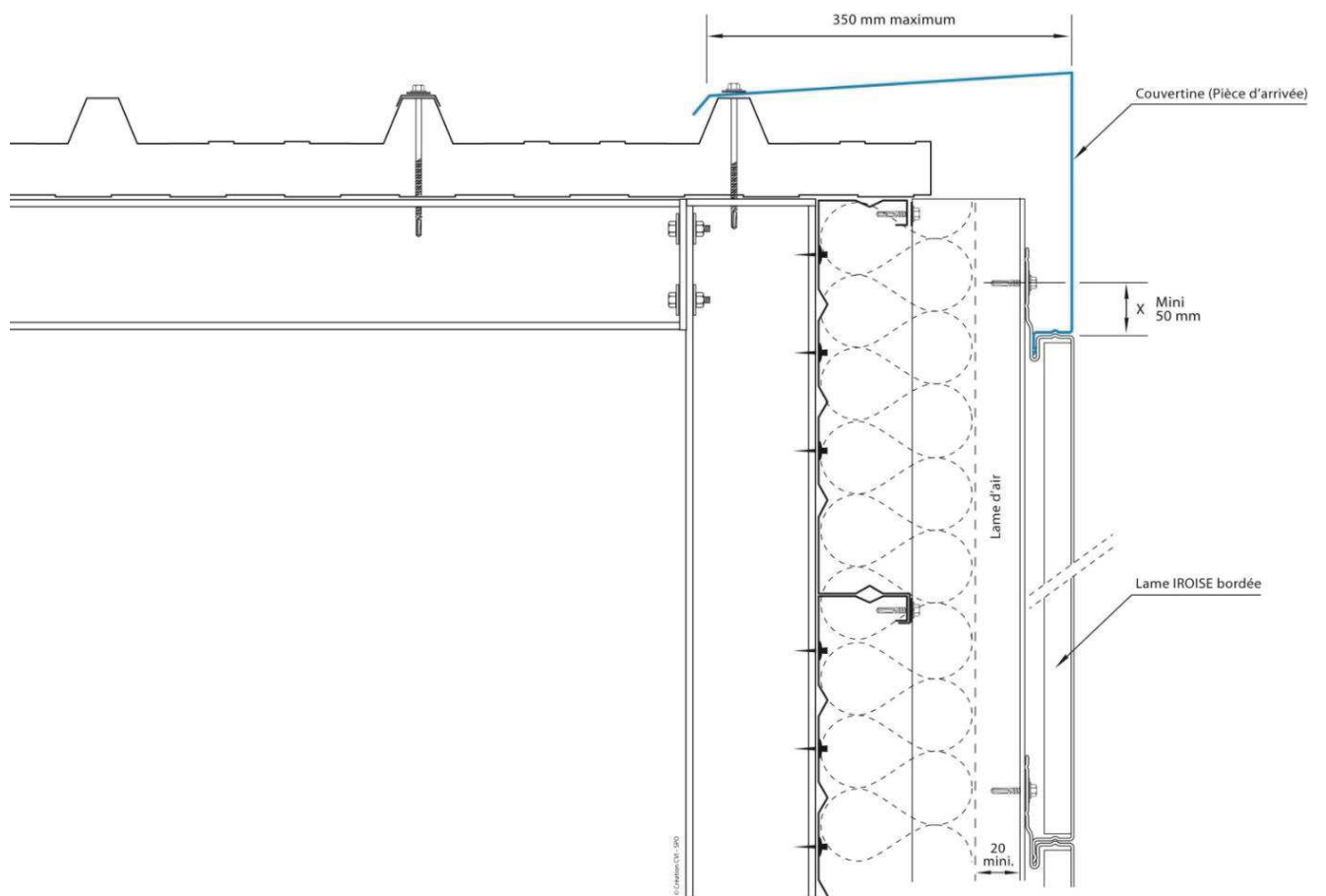
Figure 10.3 – Détail acrotère 3 Coiffe avec panneaux sandwiches
