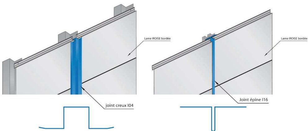
Figure 17.1 Détails joint creux vertical et joint épine, pose horizontale
