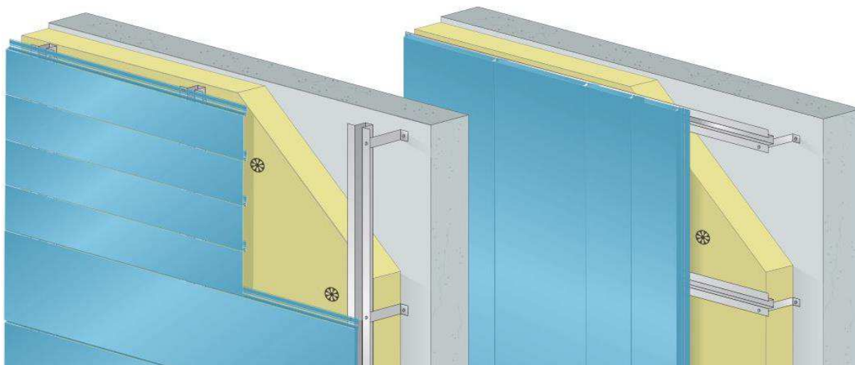
Principe de pose en bardage rapporté : bardage horizontal à gauche et bardage vertical à droite
