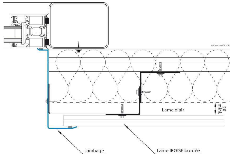
Figure 15 – Détails jambage pose verticale
