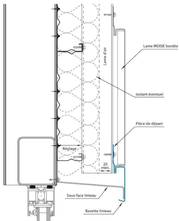
Figure 14.3 – Détails linteaux (pose en double peau)
