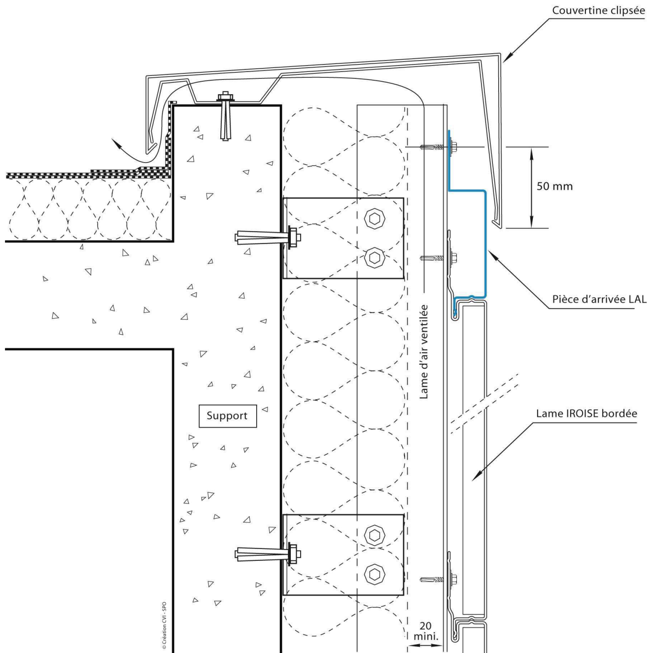
Figure 10.1 – Détail acrotère 1 LAL et ventilation haute
