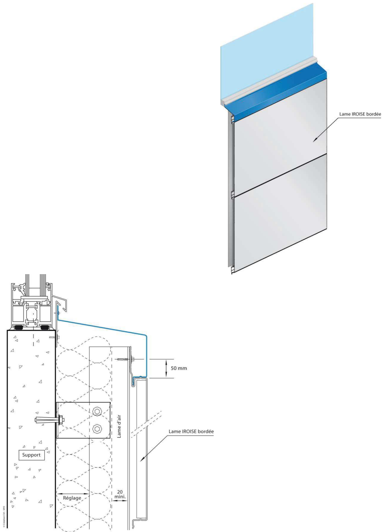
Figure 13 – Détail appui 2
