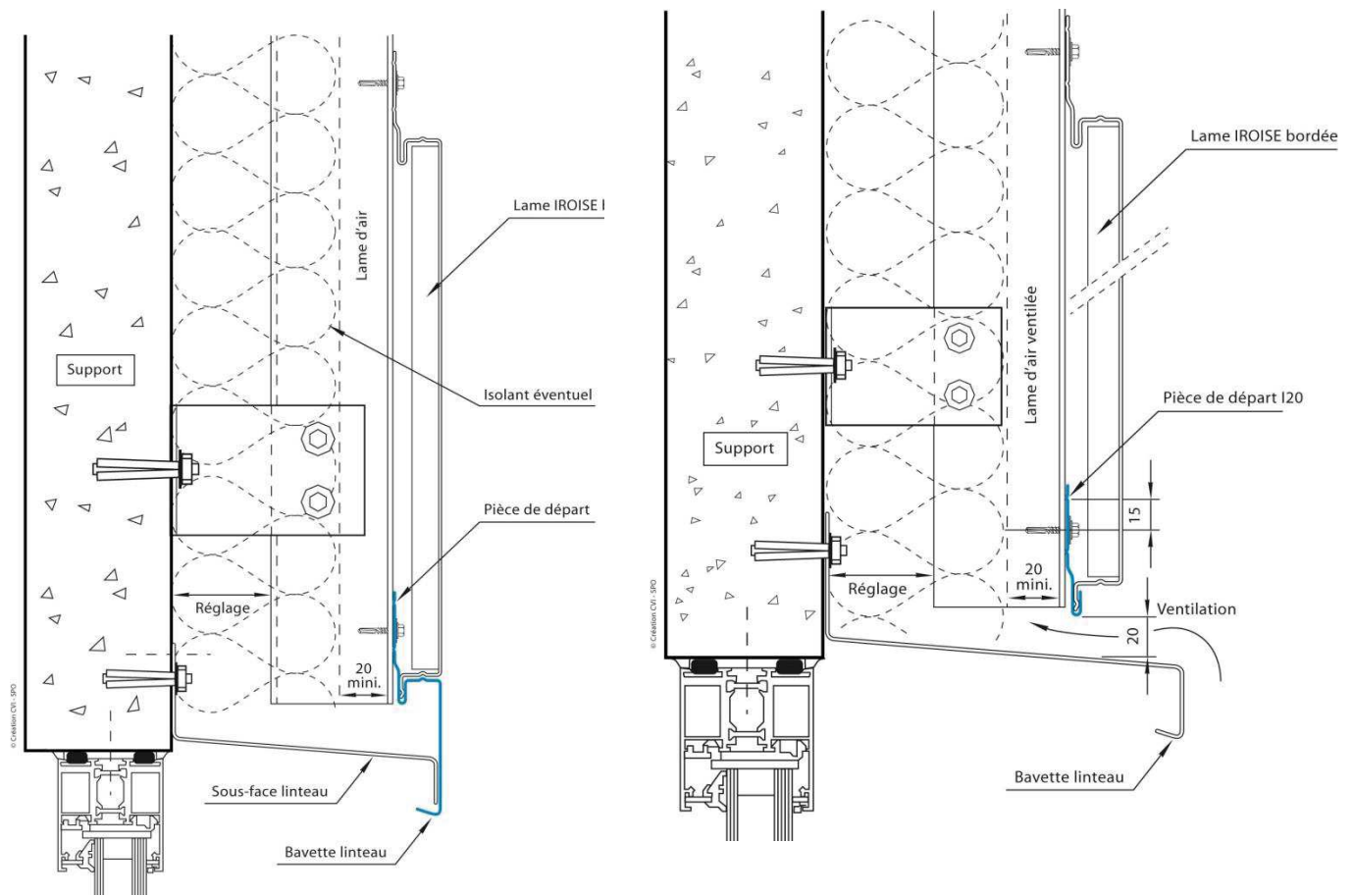
Figure 14.1 et 14.2 – Détails linteaux I20 (pose rapportée)
