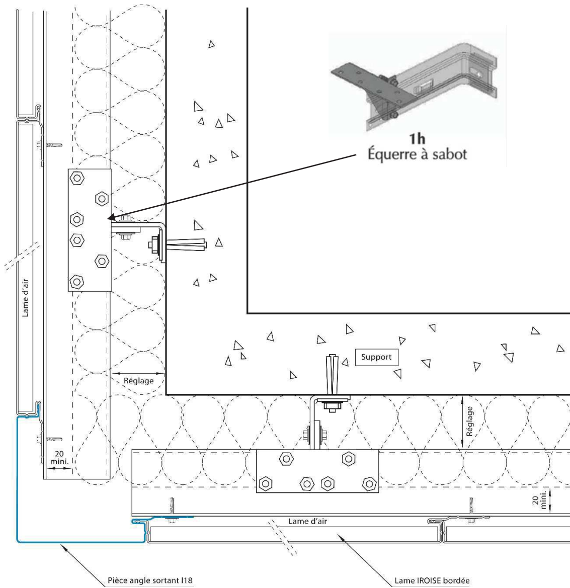
Figure 23 – Détail angle sortant pose verticale
