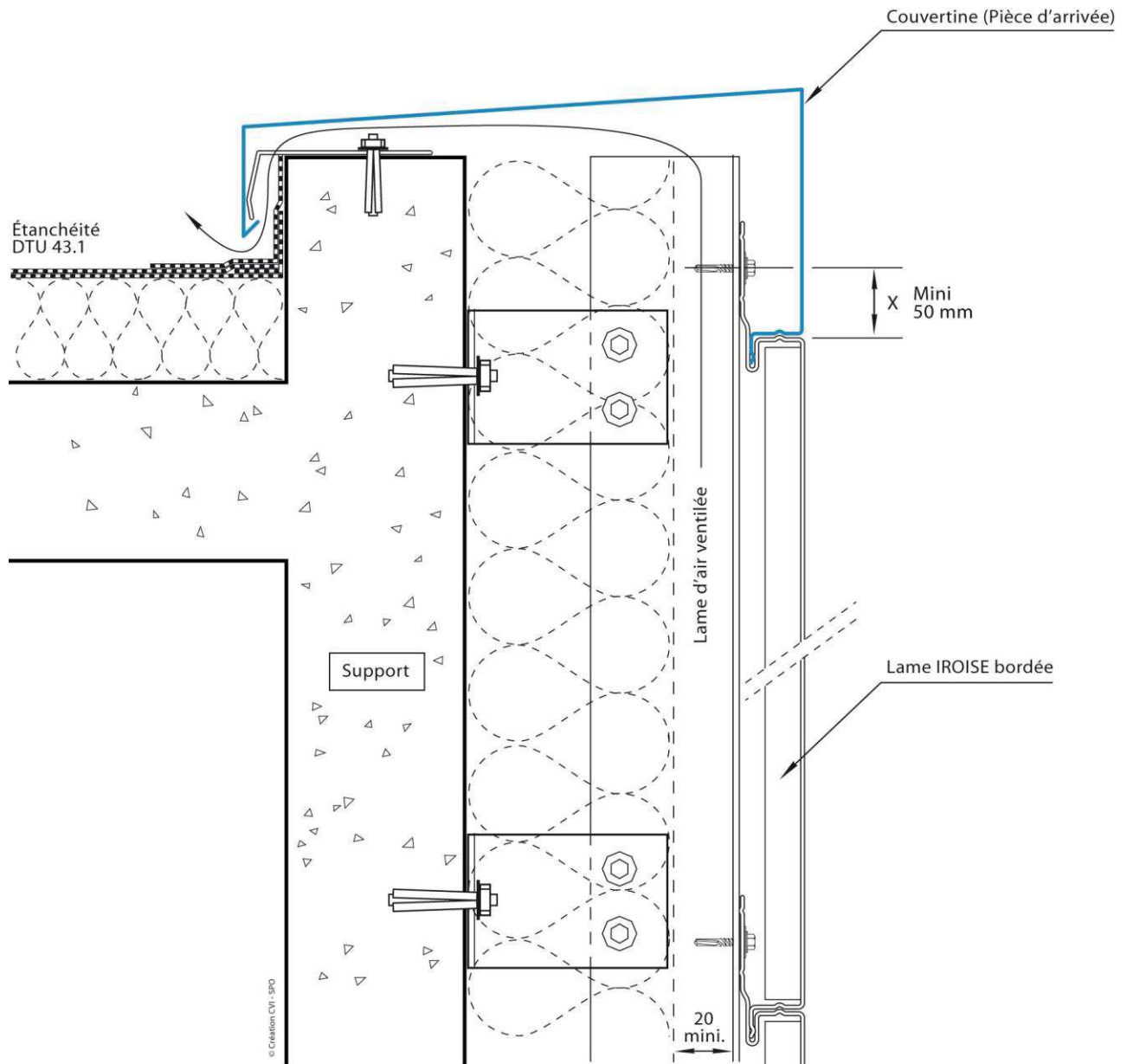
Figure 10.2 – Détail acrotère 2 Coiffe
