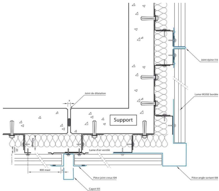
Figure 17 – Détails angle sortant
