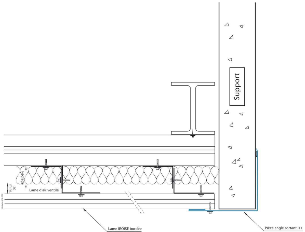
Figure 19 – Détails angle sortant simple
