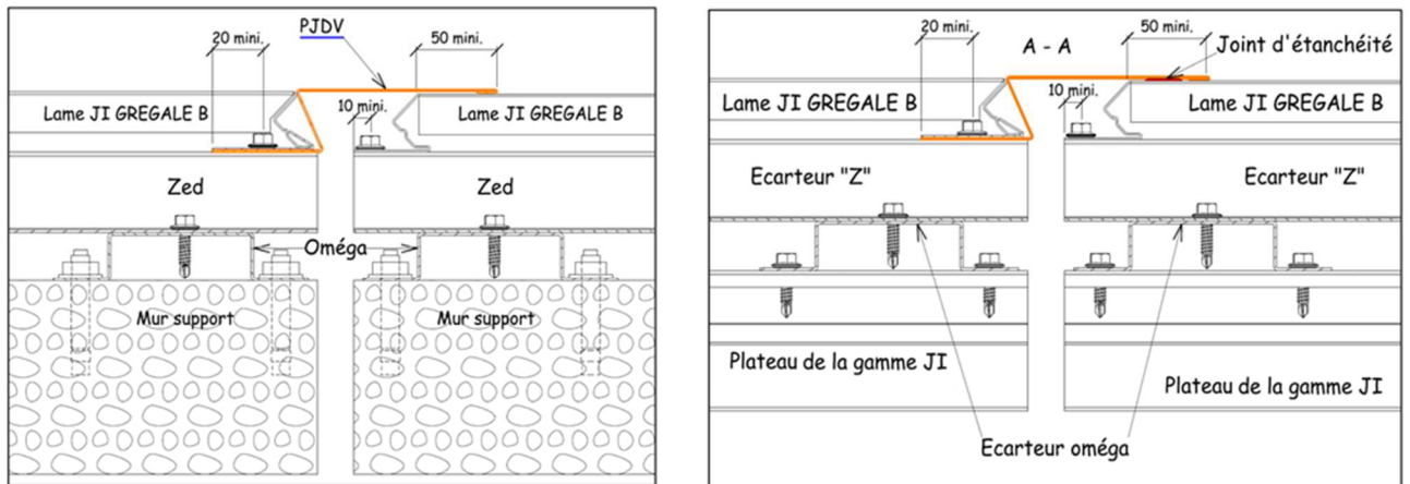
Figure 58 - Joint de dilatation en pose verticale, référence PJDV
