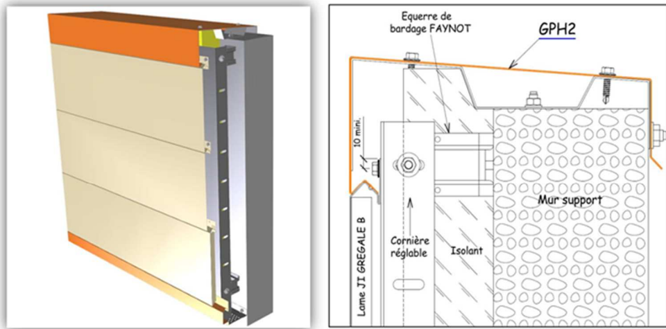
Figure 28 – Coiffe d'acrotère GPH2
