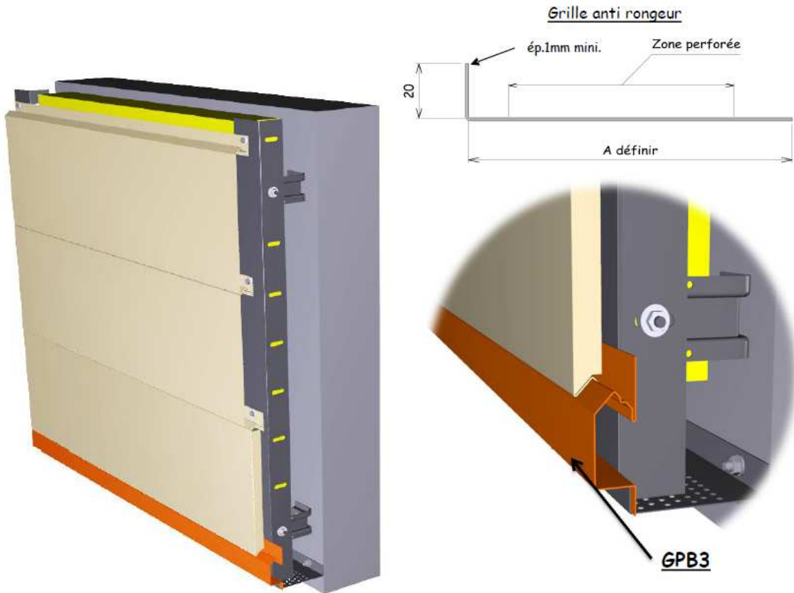
Figure 25 - Pièce de départ GPB3
