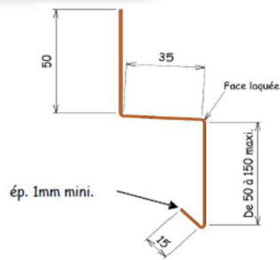
Figure 27 - Pièce de fin GPH1
