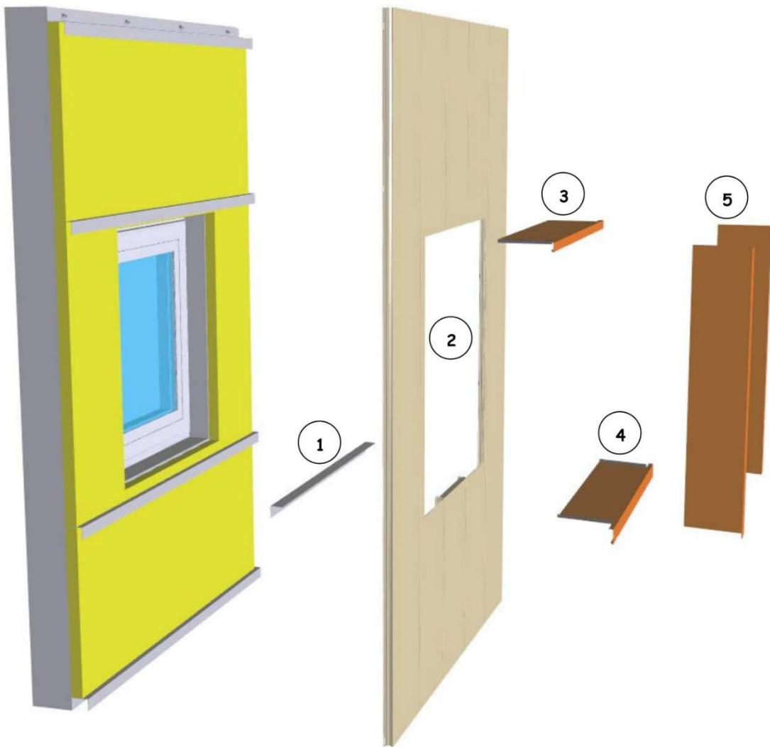
Figure 47 - Habillage de baie en pose verticale de bardage rapporté
