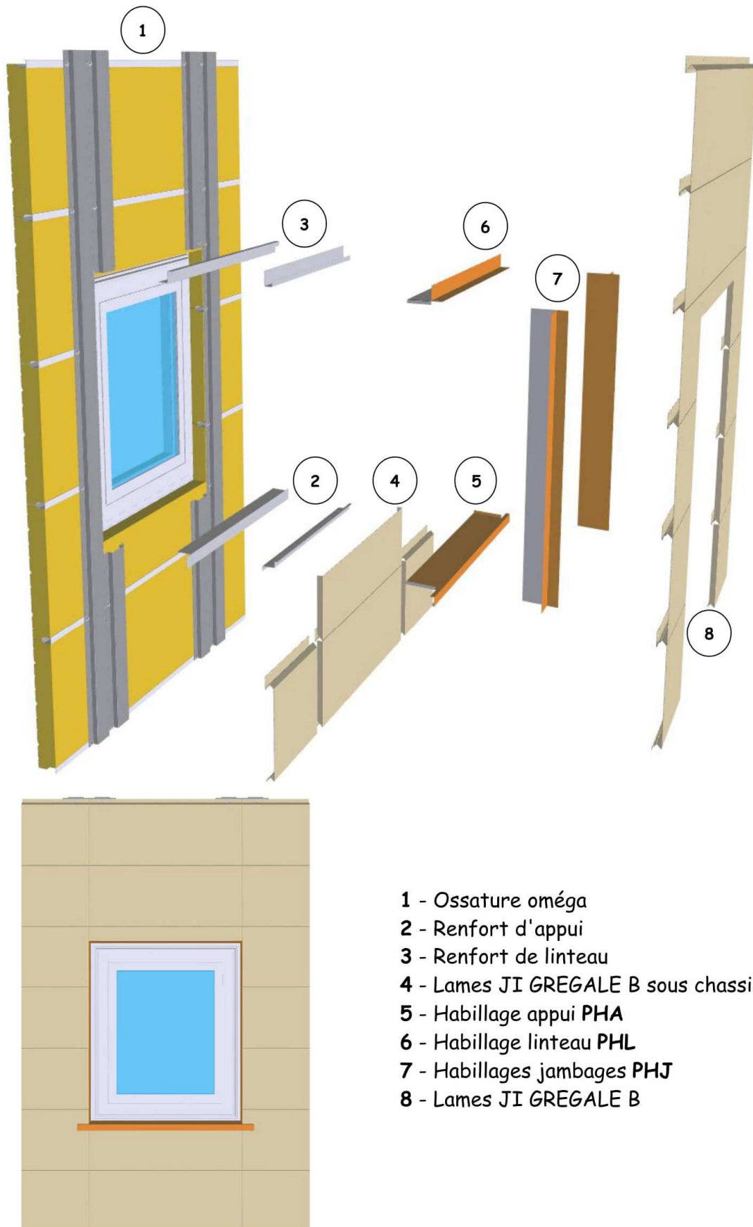
Figure 43 – Habillage de baie en pose horizontale en bardage double peau sur plateaux
