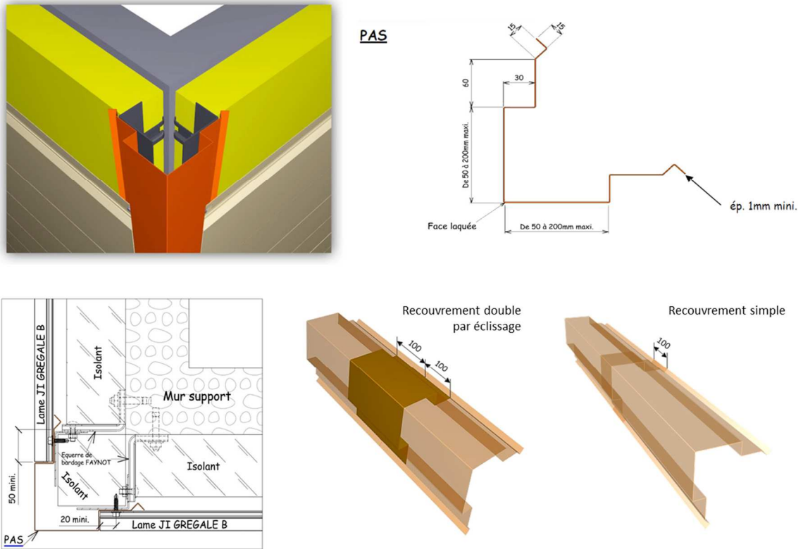
Figure 38 - Angle sortant - Référence PAS
