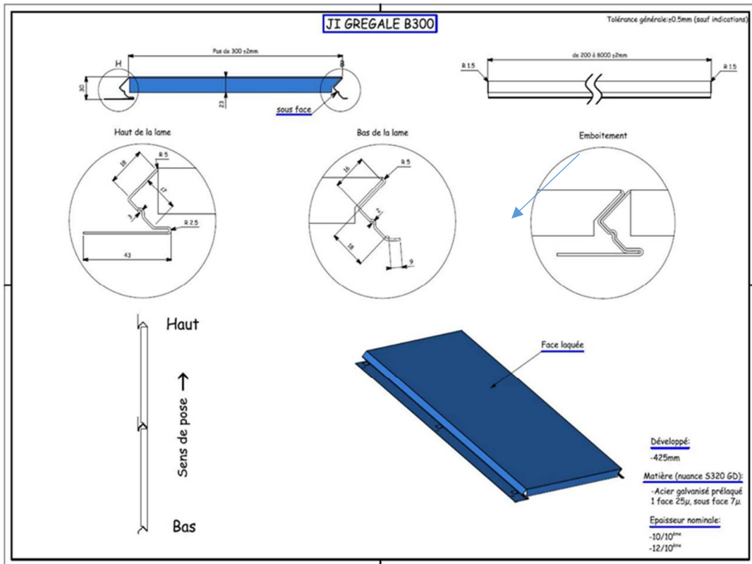
Figure 1 - Géométrie de la lame Grégale B300 SC.
