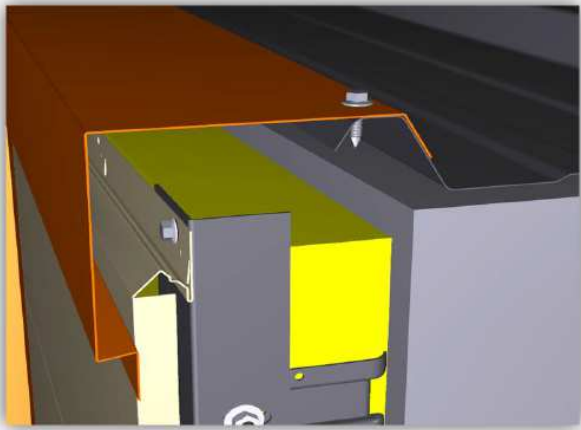
Figure 31 - Rive de couverture - liaison avec le haut de bardage, référence BR
