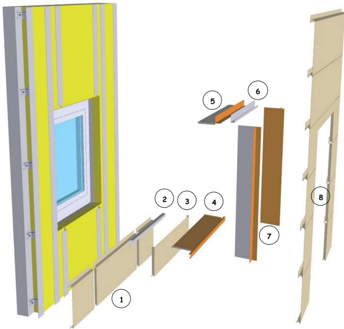
Figure 44 – Habillage de baie en pose horizontale de bardage rapporté
