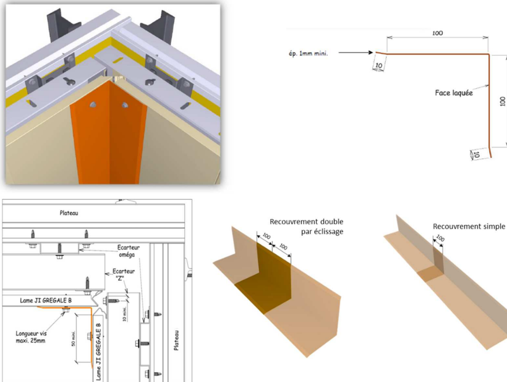
Figure 36 - Angle rentrant en pose verticale, référence AR
