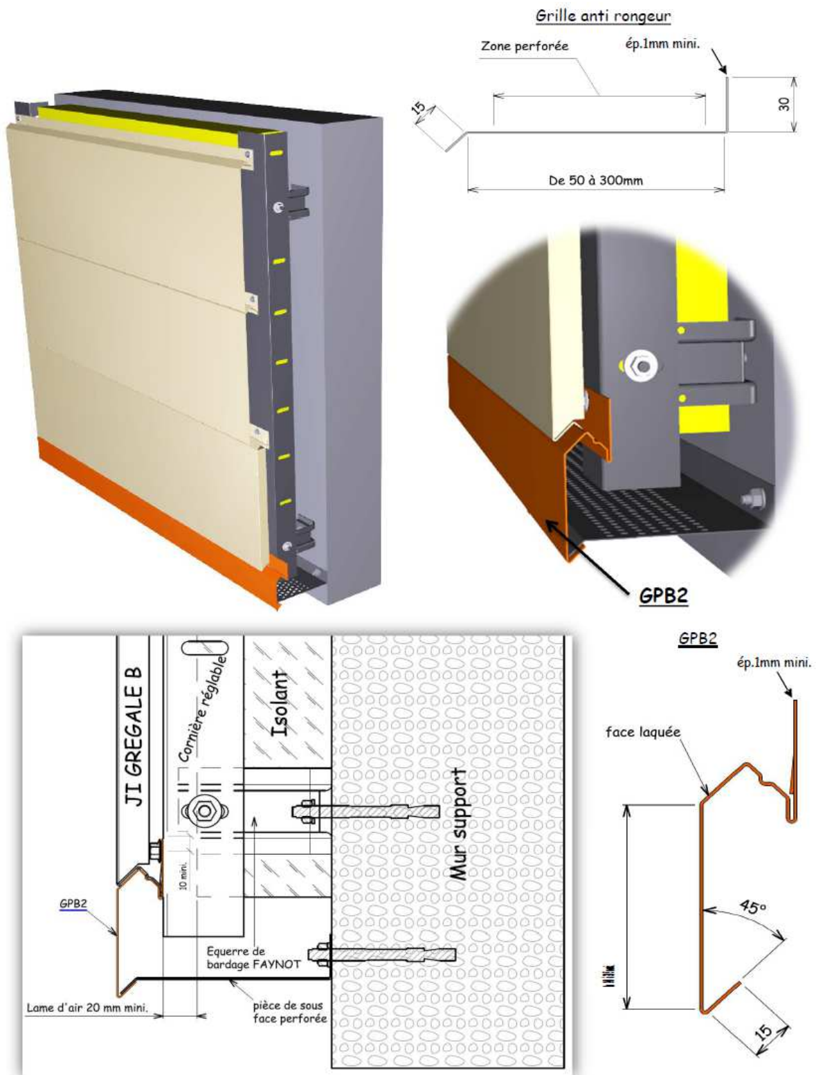
Figure 24 - Pièce de départ GPB2
