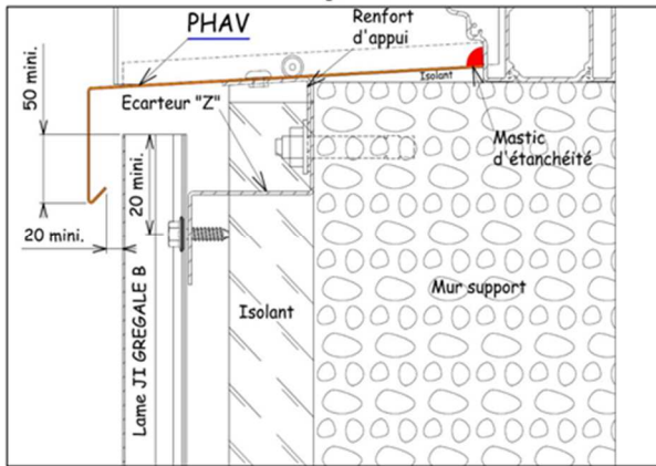
Figure 52 - Appui bas d'habillage de baie en pose verticale des lames, référence PHAV
