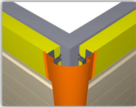
Figure 40 - Angle sortant cintré - Référence PASC
