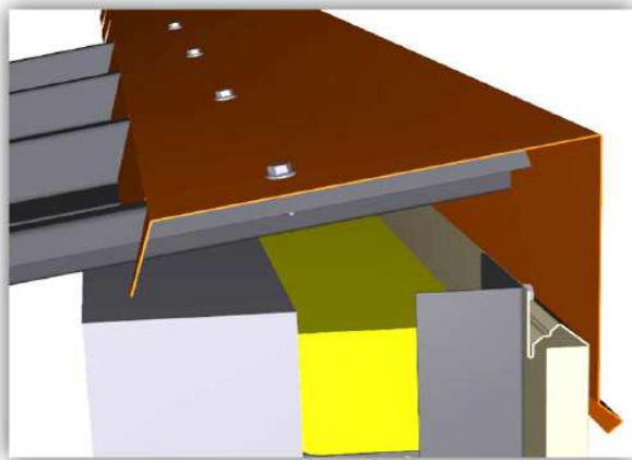
Figure 30 - Faîtage sur mur de façade, référence BF
