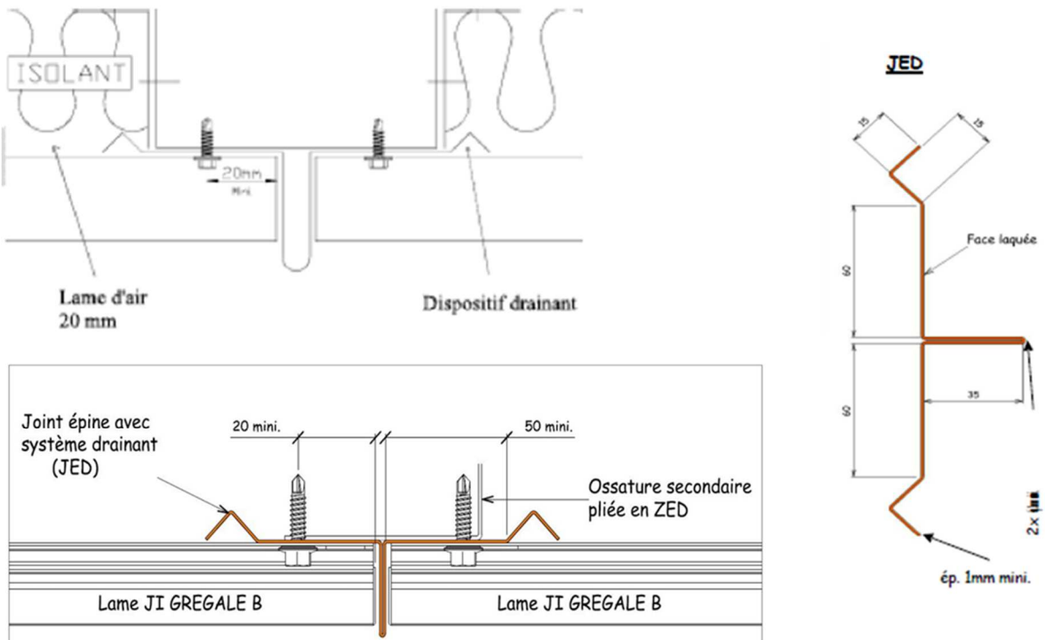
Figure 33 - Joint en épine - Référence JE et JED "Drainant"
