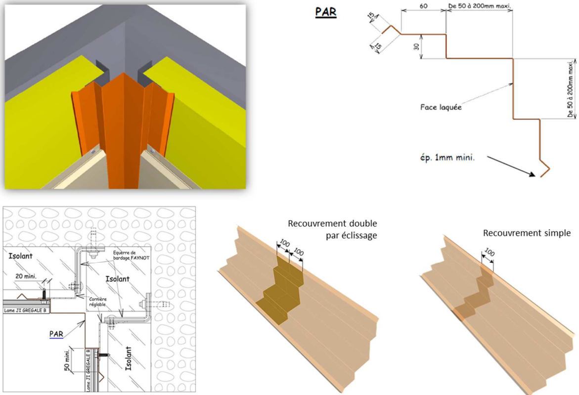
Figure 35 - Angle rentrant - Référence PAR
