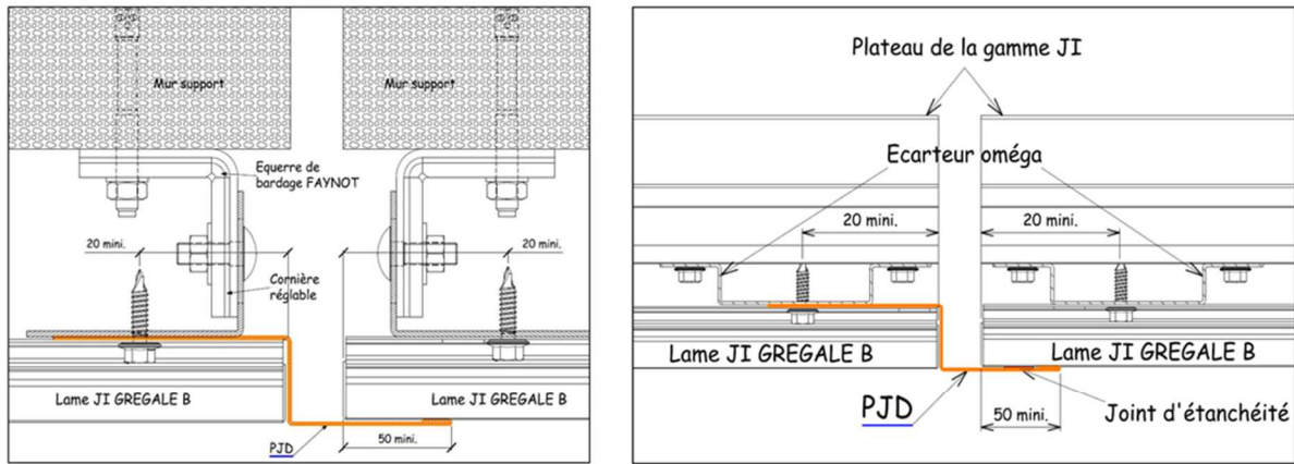
Figure 57 - Joint de dilatation en pose horizontale, référence PJD
