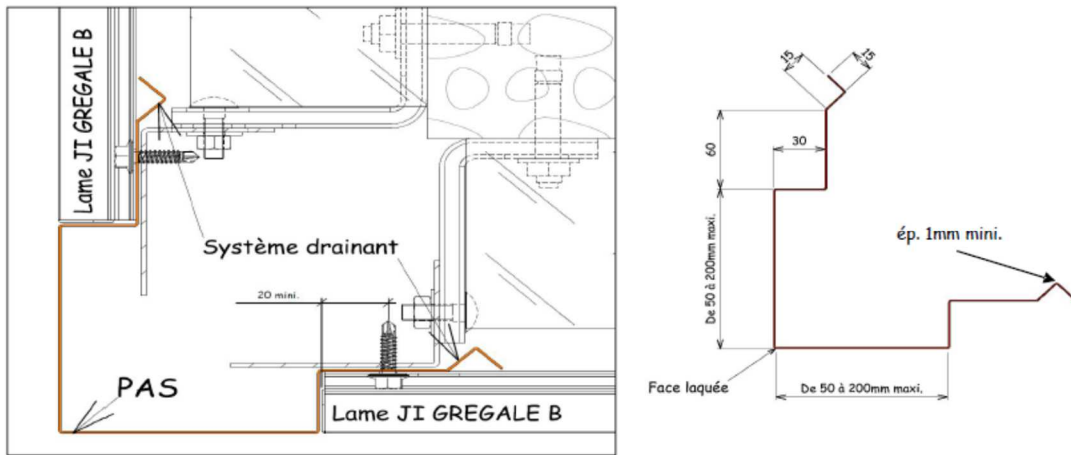
Figure 22 - Pièce drainant d'angle, référence PAS
