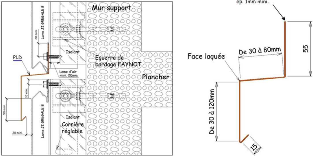
Figure 55 - Nez de plancher – Pièce larmier, référence PLD, pour pose horizontale des lames
