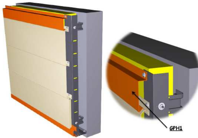
Figure 27 - Pièce de fin GPH1
