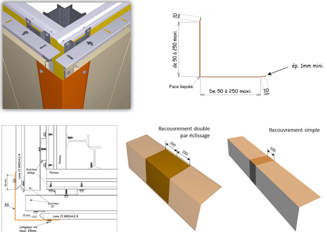
Figure 39 - Angle sortant en pose verticale, référence AS
