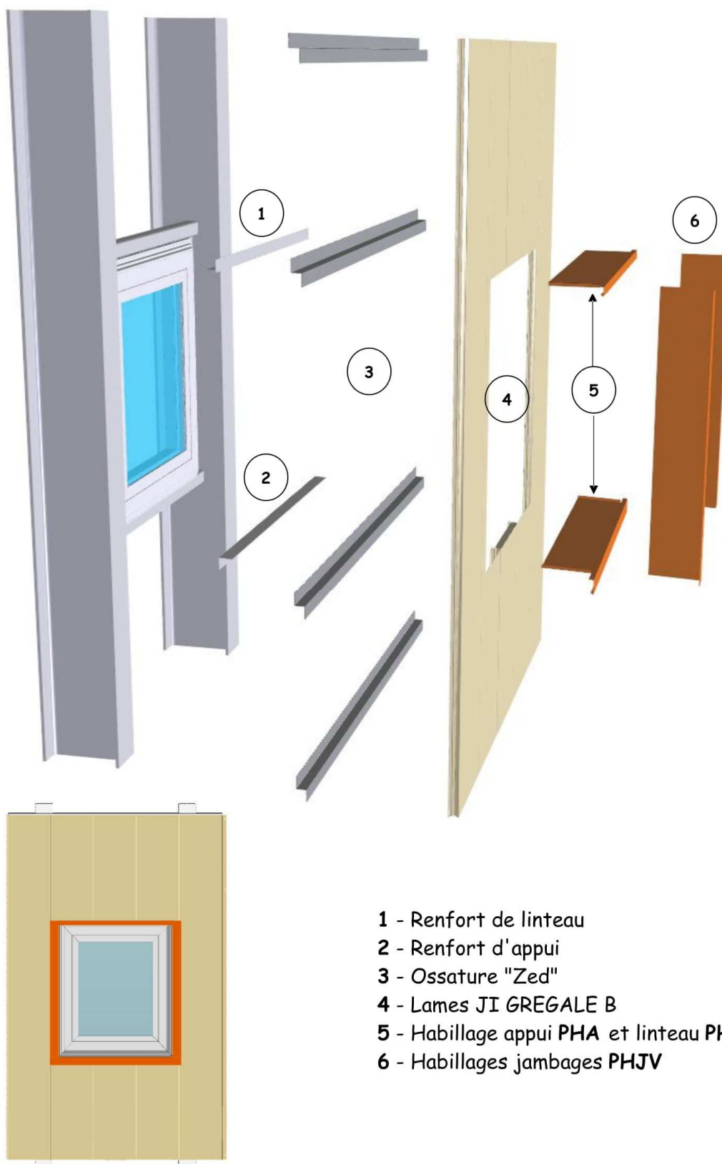
Figure 48 - Habillage de baie en pose verticale de bardage simple peau
