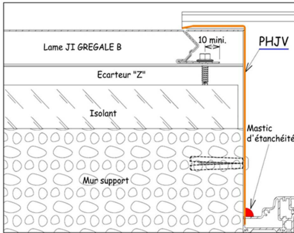
Figure 53 - Jambage pour habillage de baie en pose verticale des lames, référence PHJV
