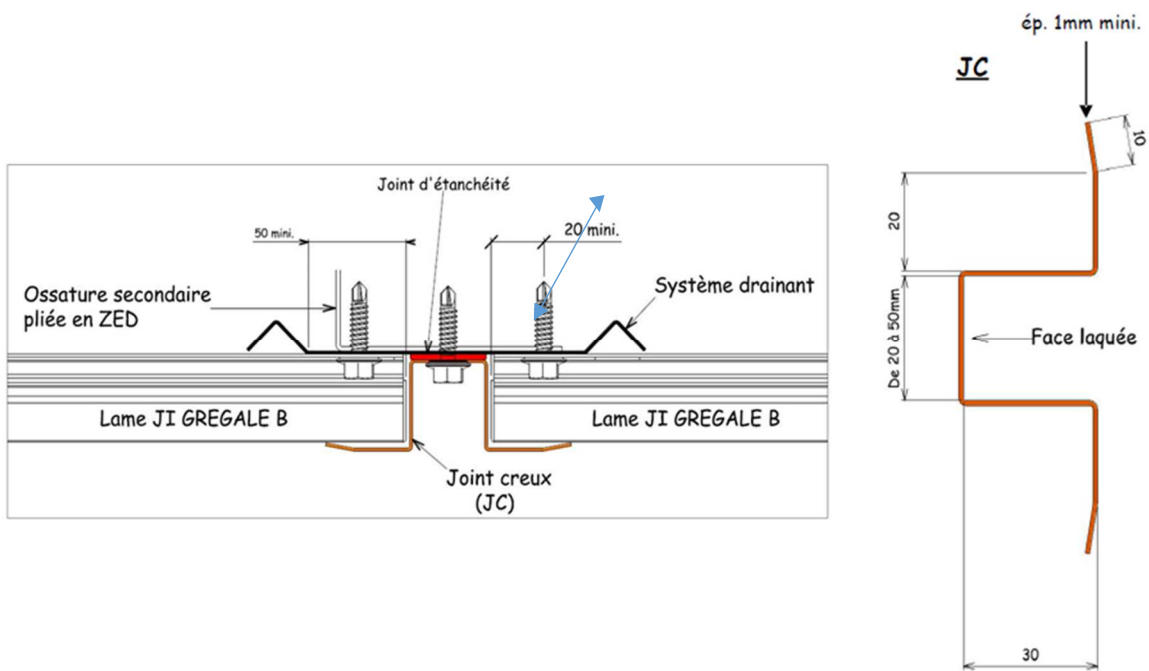
Figure 32 - Joint creux - Référence JC
