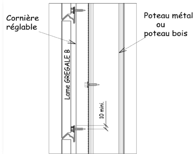
Figure 6 - Principe de pose en bardage horizontal simple peau
