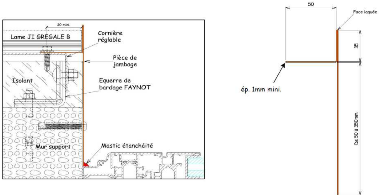
Figure 50 - Jambage pour baie, référence PHJ, pour pose horizontale des lames
