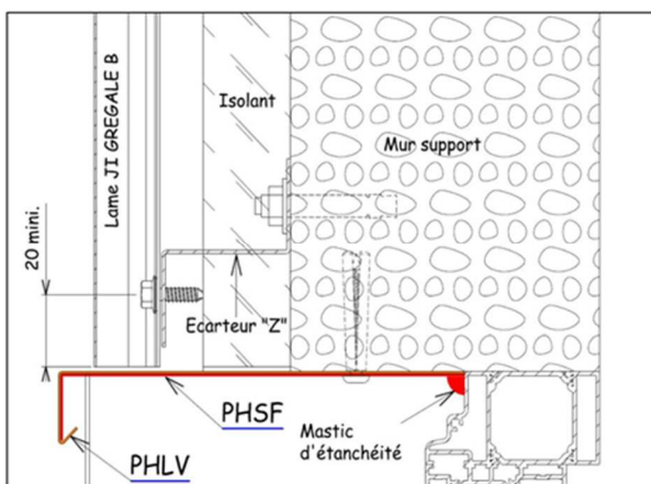
Figure 54 - Linteau pour habillage de baie en pose verticale des lames, référence PHLV
