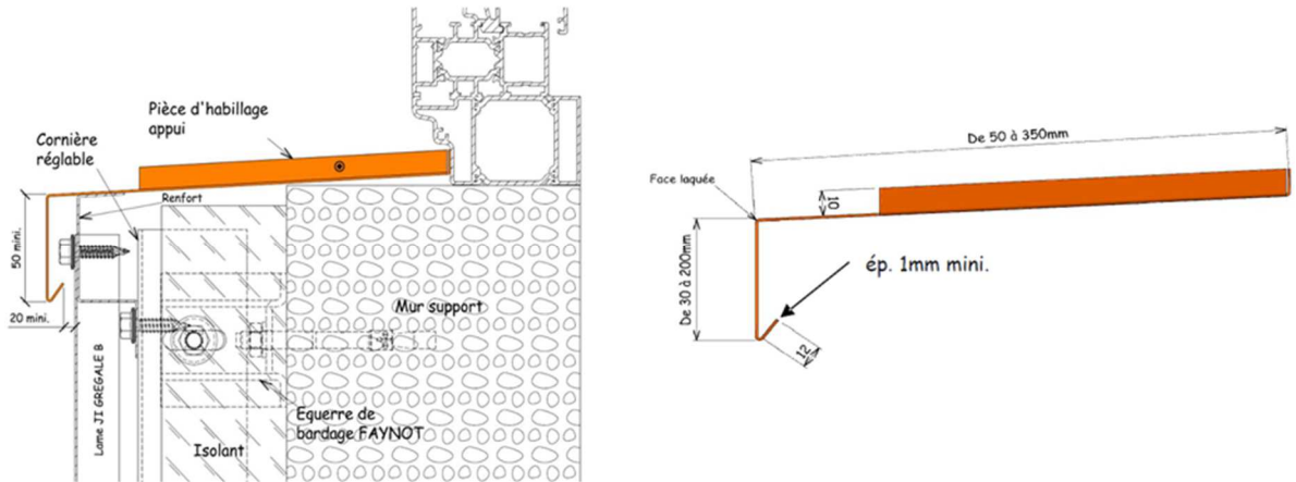
Figure 49 - Appui de baie, référence PH, pour pose horizontale des lames
