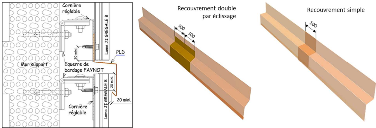
Figure 34 - Interruption du bardage avec larmier, référence PLDV
