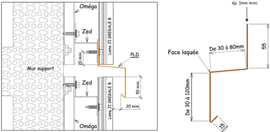
Figure 56 - Interruption du bardage avec pièces larmier, référence PLDV, pour pose verticale des lames
