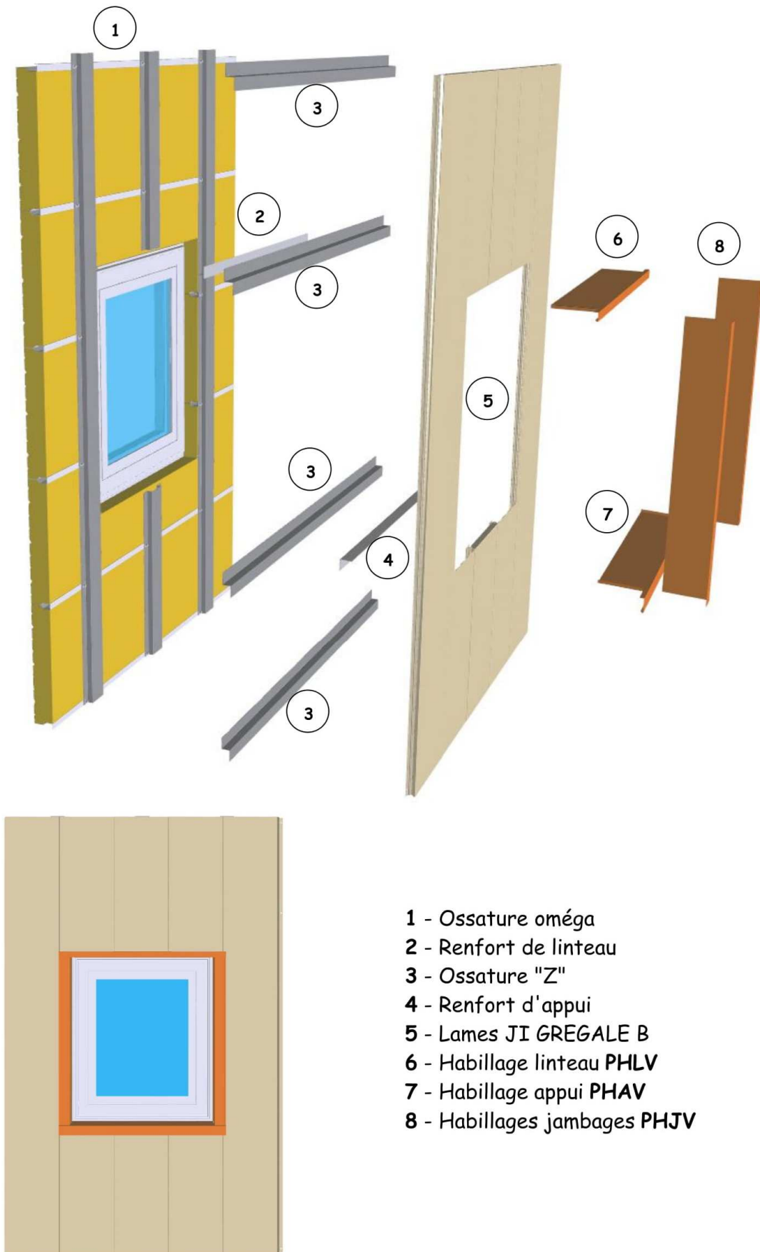
Figure 46 - Habillage de baie en pose verticale en bardage double peau sur plateaux
