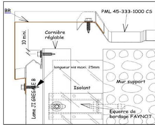
Figure 31 - Rive de couverture - liaison avec le haut de bardage, référence BR
