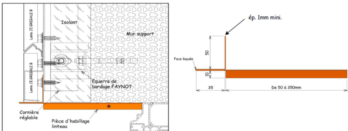
Figure 51 - Linteau pour baie, référence PHL, pour pose horizontale des lames
