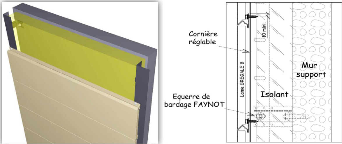
Figure 8 - Principe de pose en bardage rapporté horizontal
