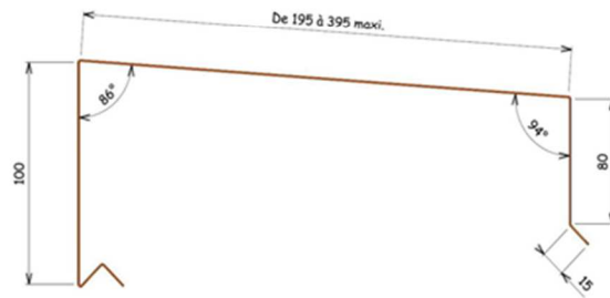
Figure 29 - Coiffe d'acrotère, référence PCA
