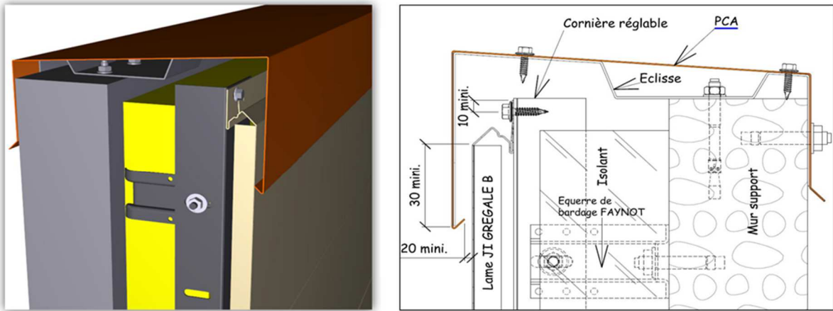
Figure 29 - Coiffe d'acrotère, référence PCA
