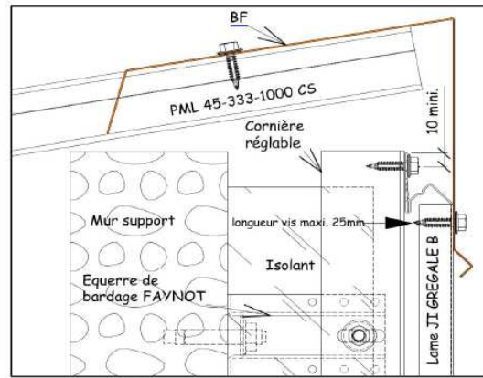
Figure 30 - Faîtage sur mur de façade, référence BF
