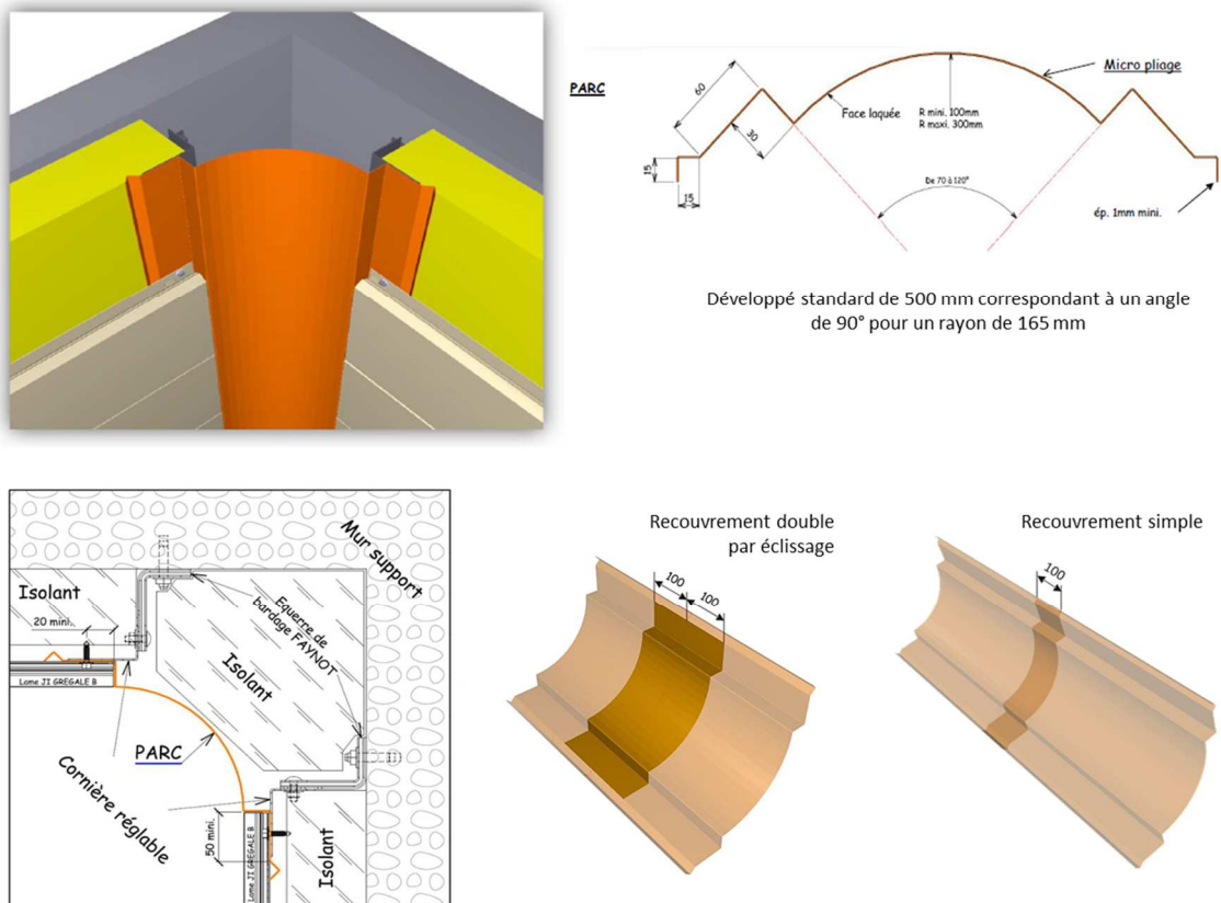
Figure 37 - Angle rentrant cintré - Référence PARC
