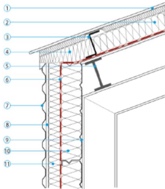
Coupe
