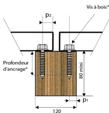
Jonction en about de plateau
