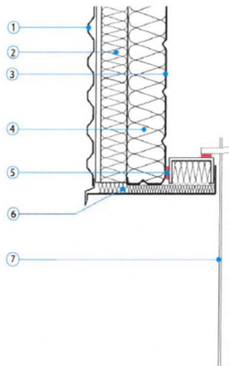
Coupe
