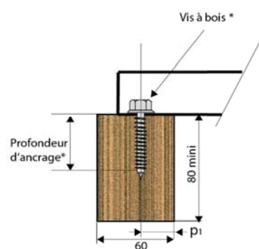
Jonction en appuis d'extrémité
