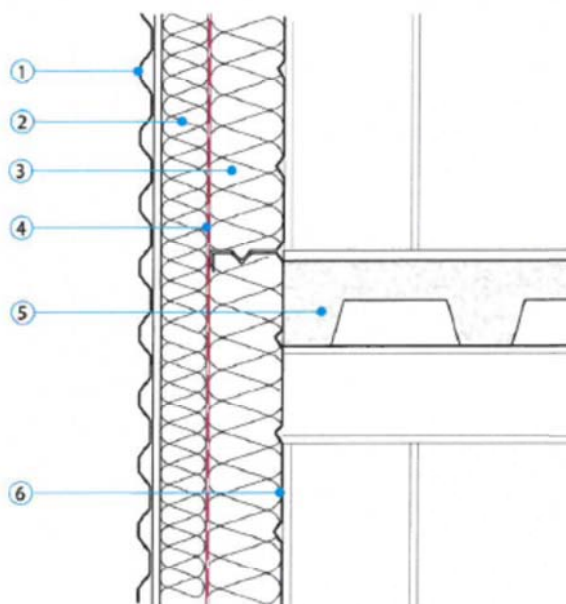
Coupe
