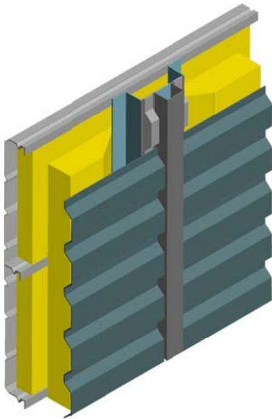
Hauteur bâtiment \leq 20 m
