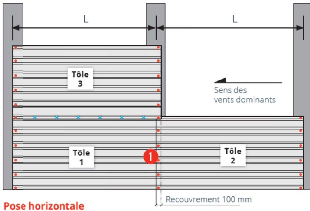
Elévation
