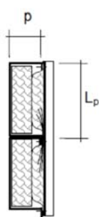
Isolant en 2 couches
